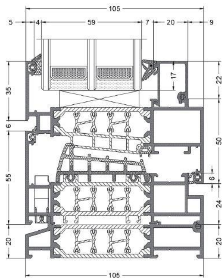
CAD断面尺寸
