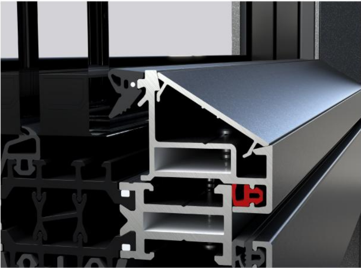
「组角压线内嵌胶条」
