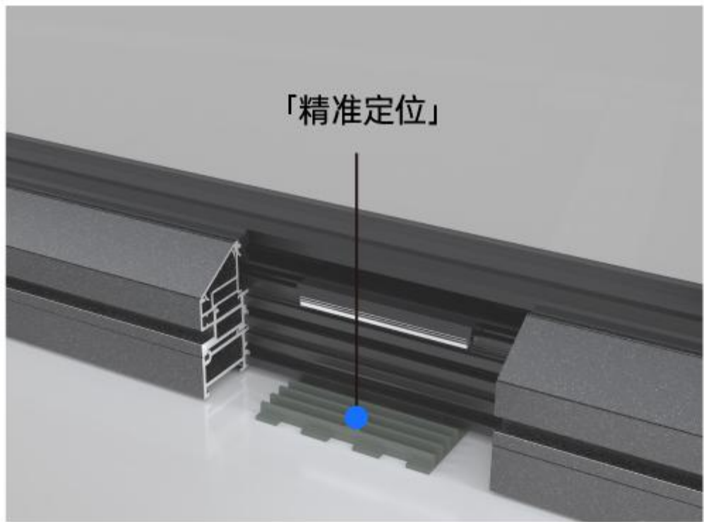
「安装辅助提示垫片」
