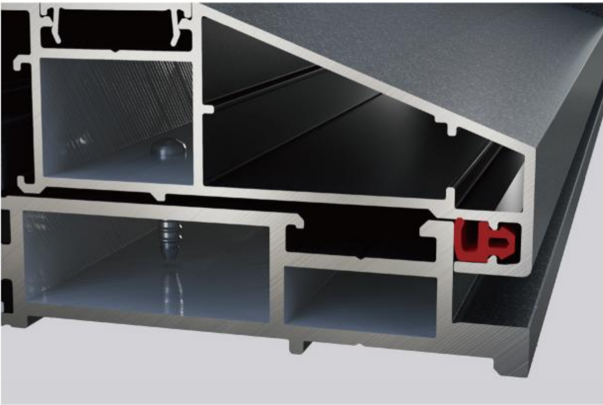
「组角压线内嵌胶条」
