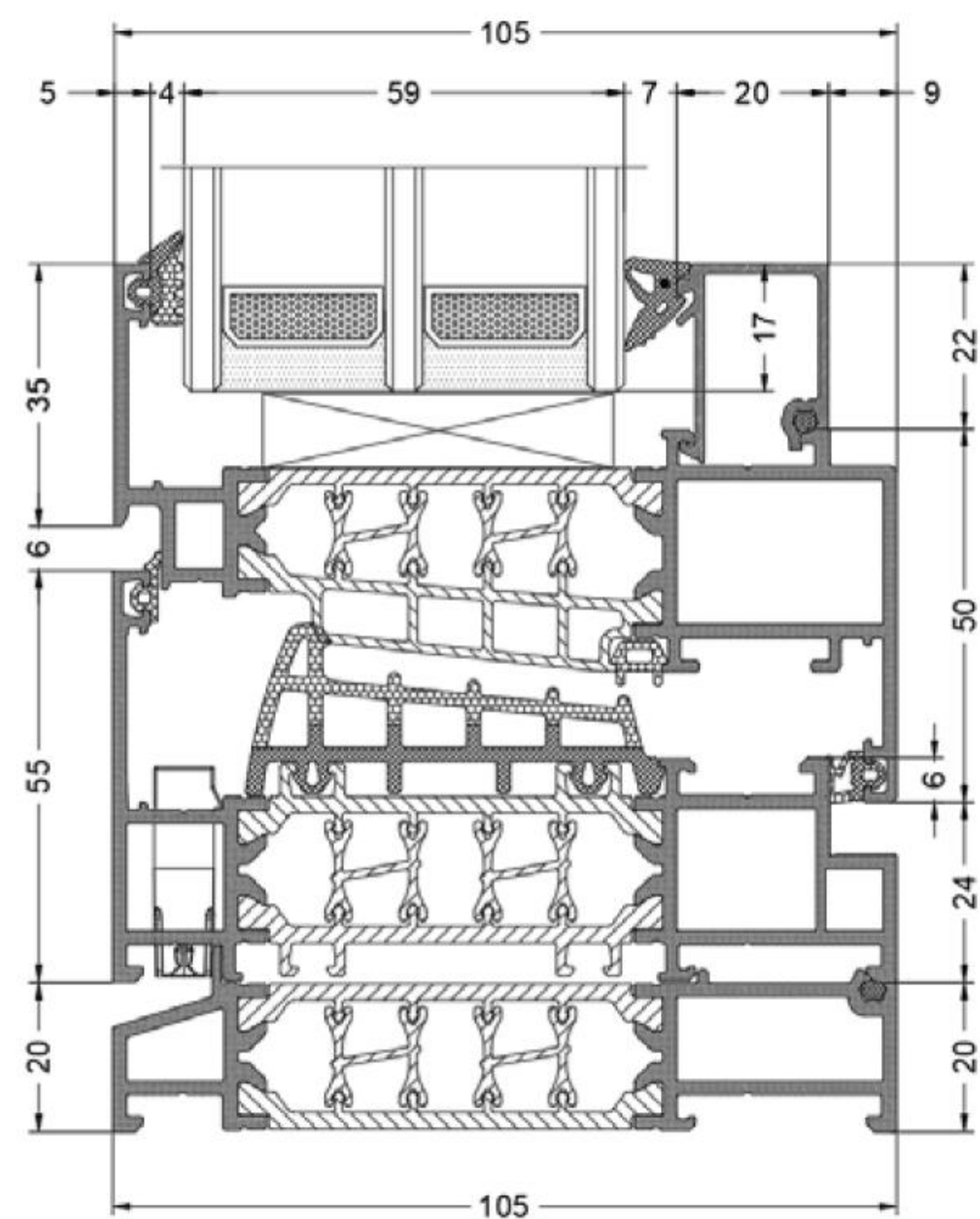
CAD断面尺寸
