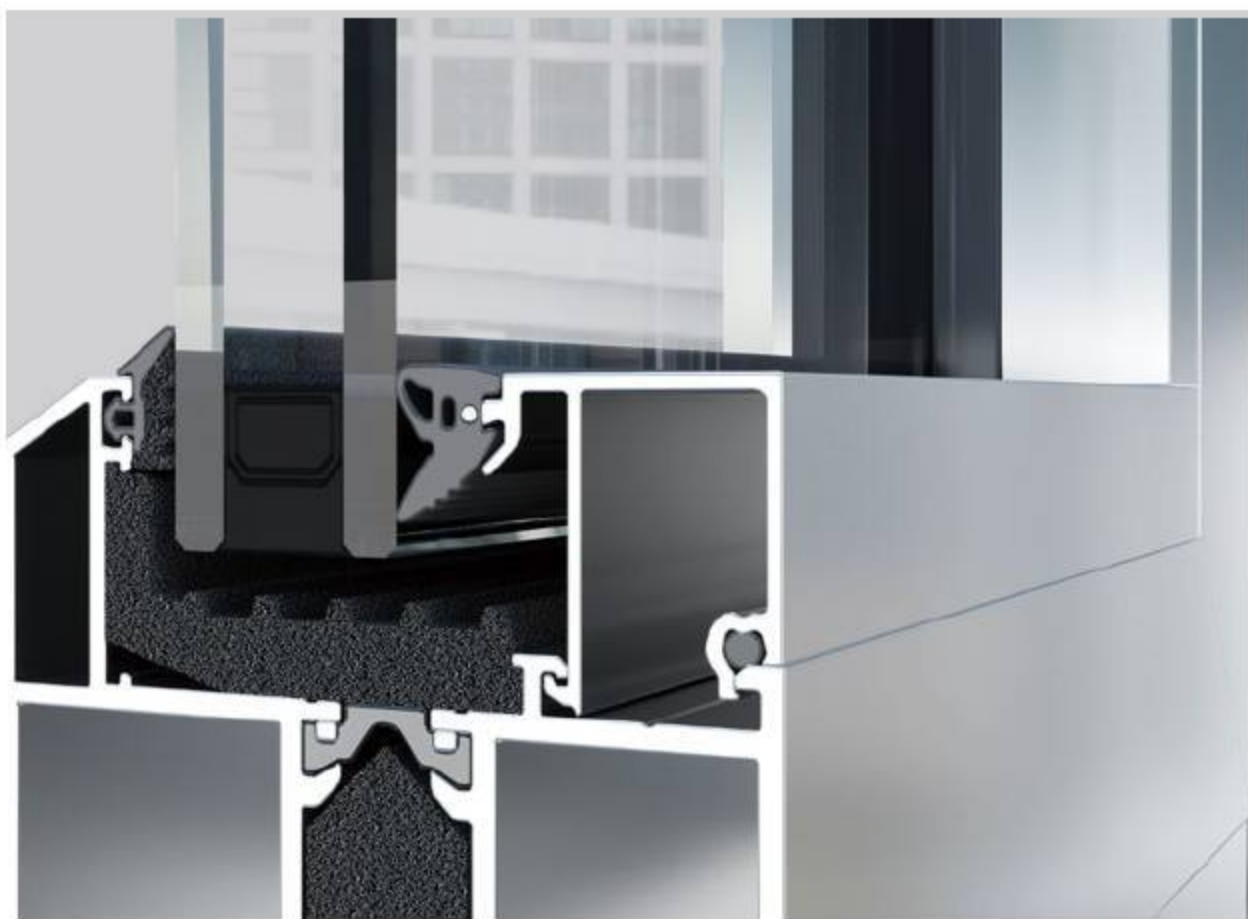
「防脱压线」
