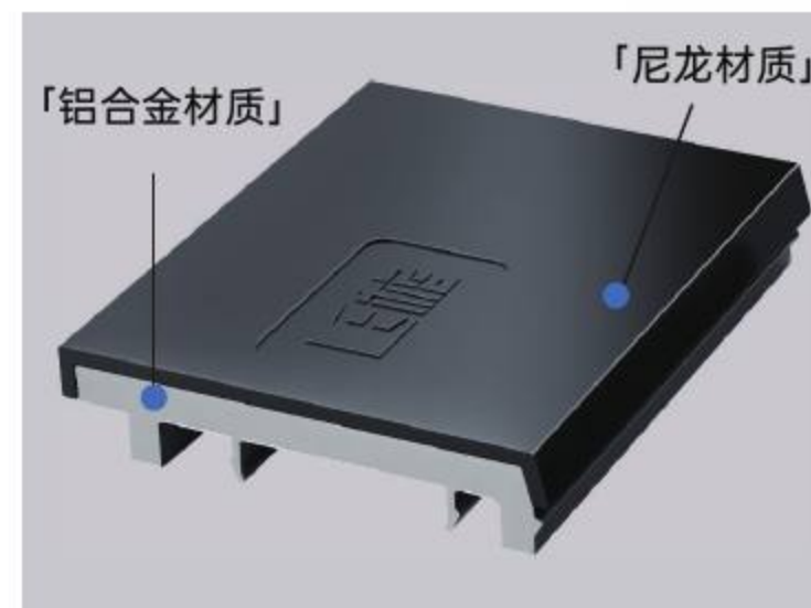
「铝合金玻璃垫块」
