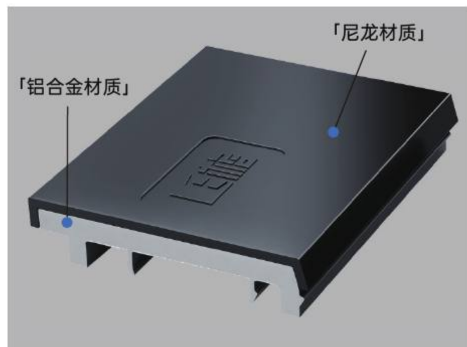
「铝合金玻璃垫块」
