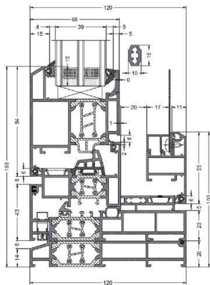
CAD断面尺寸
