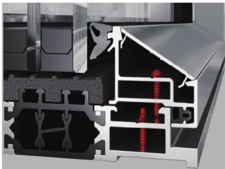
「组角压线」
