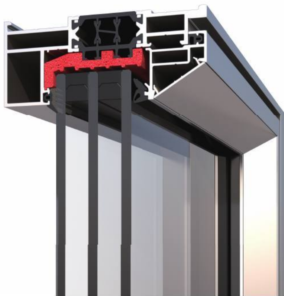
「玻璃垫棉」
