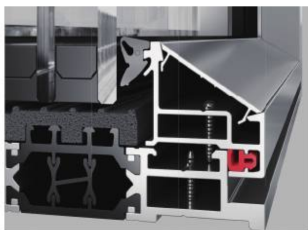
「组角压线内嵌胶条」
