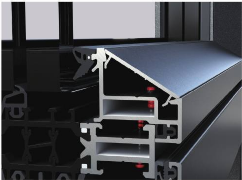
「组角压线内嵌胶条」
