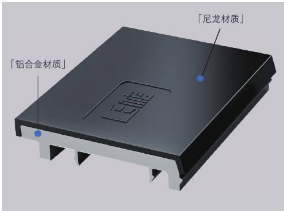
「铝合金玻璃垫块」
