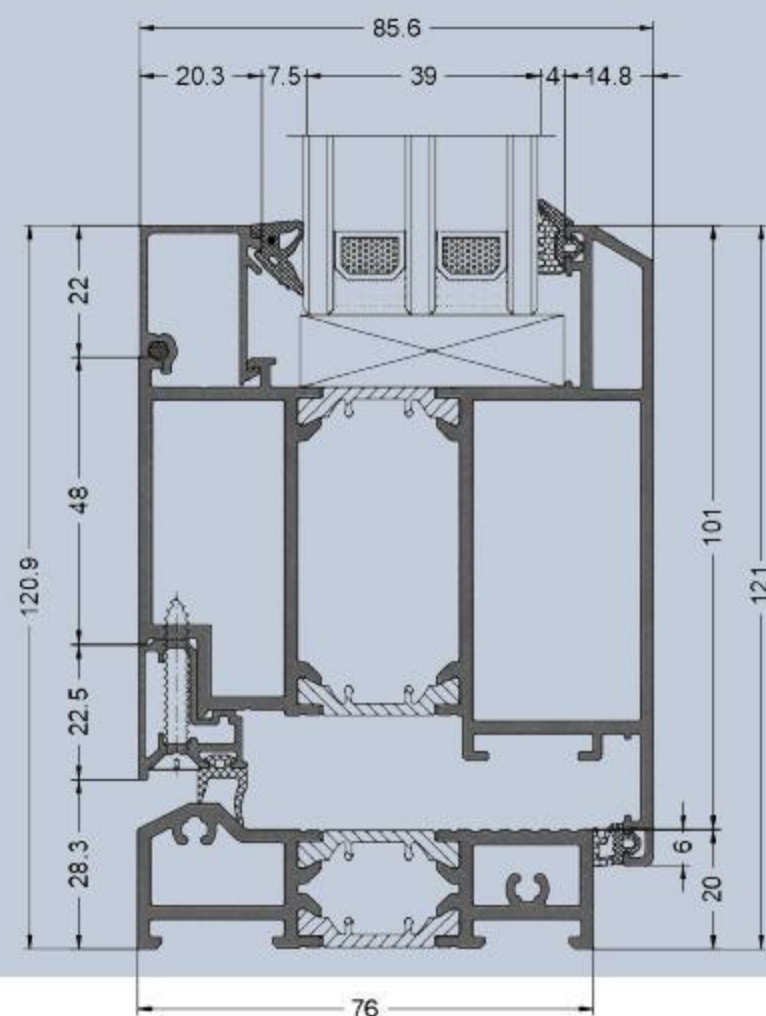
CAD 断面尺寸(外开门)
