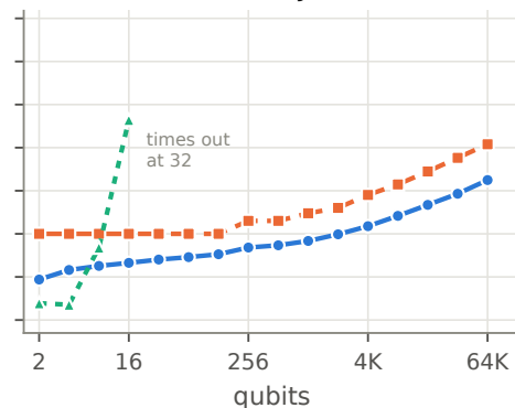
Deutsch-Jozsa
