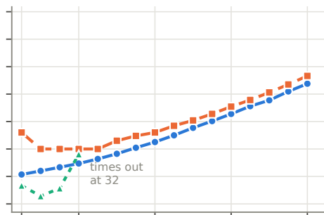
Bernstein-Vazirani
