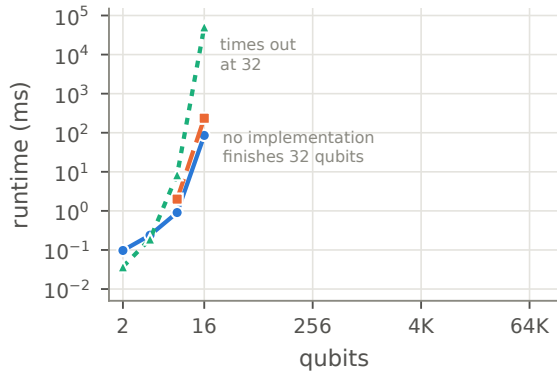
QFT
