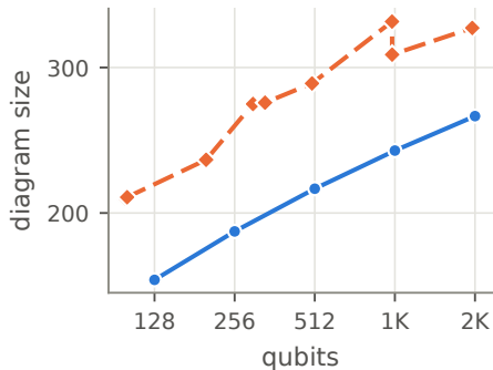
GHZ
