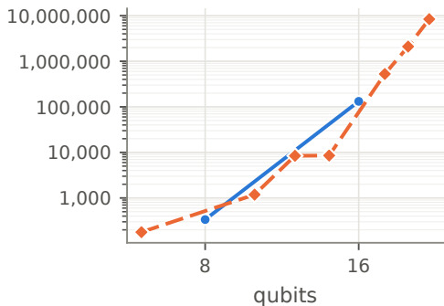
QFT
