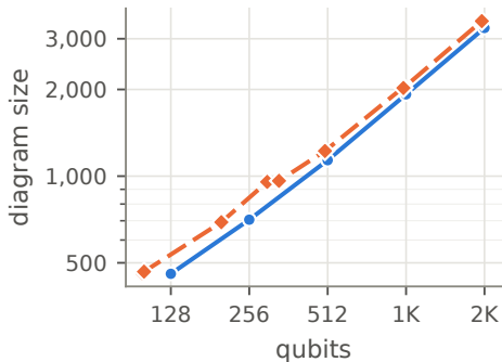
Bernstein-Vazirani
