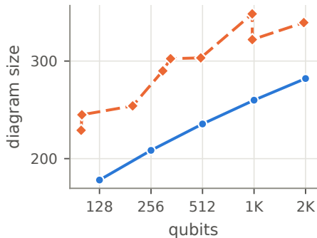
Deutsch-Jozsa
