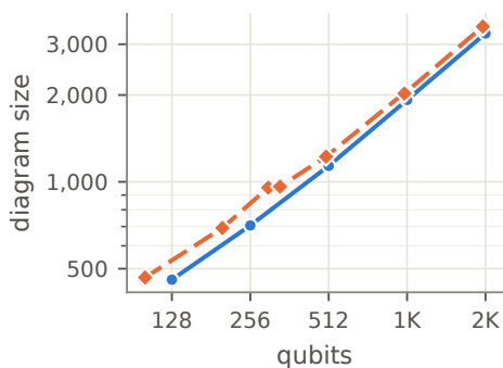
Bernstein-Vazirani
