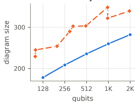
Deutsch-Jozsa
