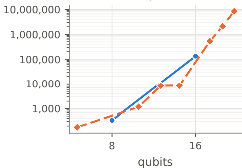
QFT
