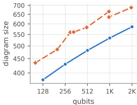
GHZ
