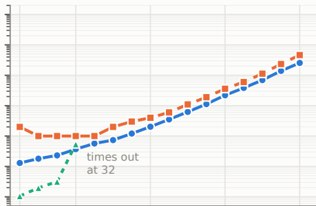
Bernstein-Vazirani
