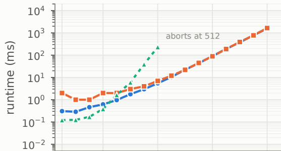
GHZ
