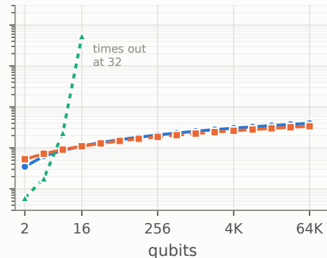
Deutsch-Jozsa
