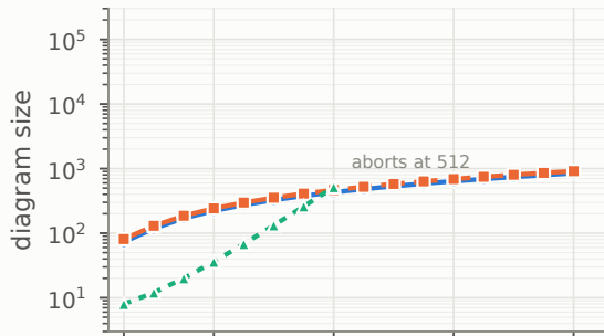
GHZ
