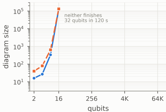
QFT
