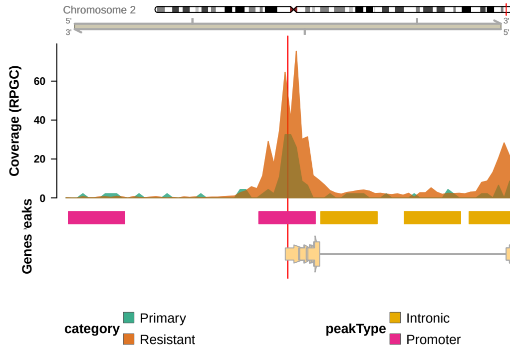
rs35277801 (UBE2F),Promoter (&lt;=1kb)
