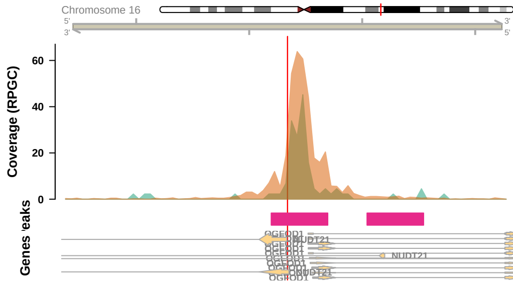
rs75289223 (NUDT21),Promoter (&lt;=1kb)
