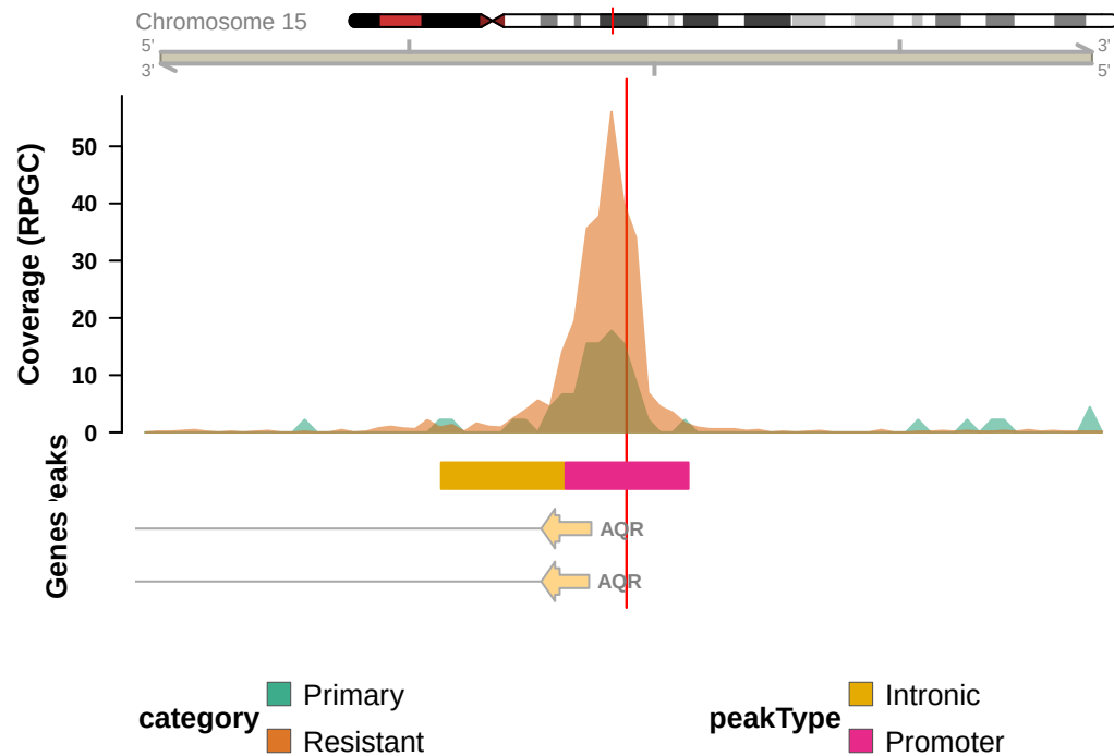
rs7164266 (AQR),Promoter (&lt;=1kb)
