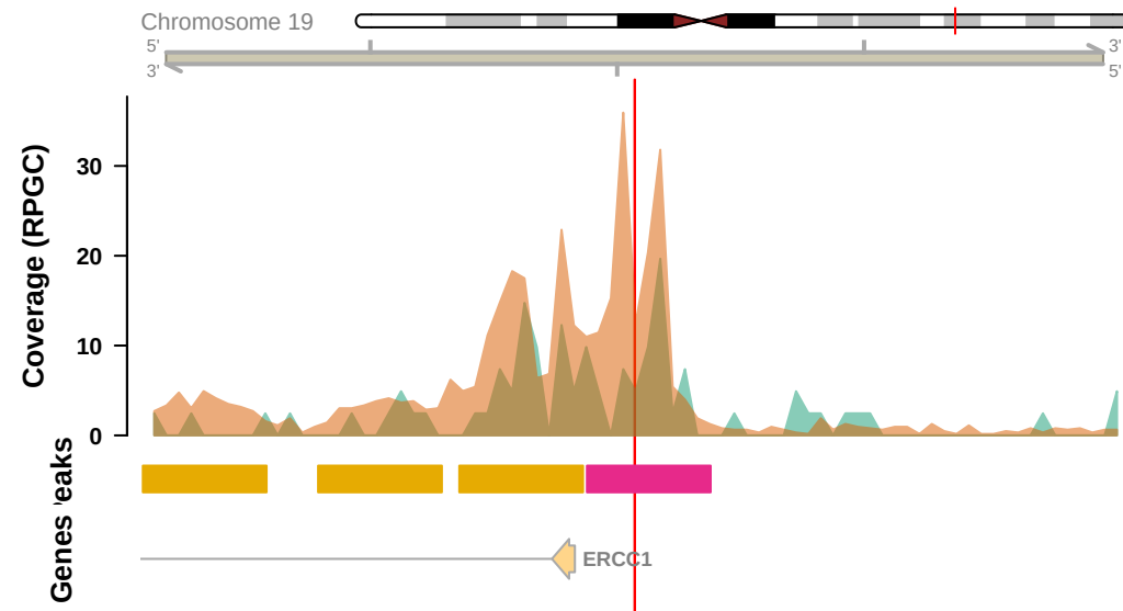
rs150652488 (ERCC1),Promoter (&lt;=1kb)
