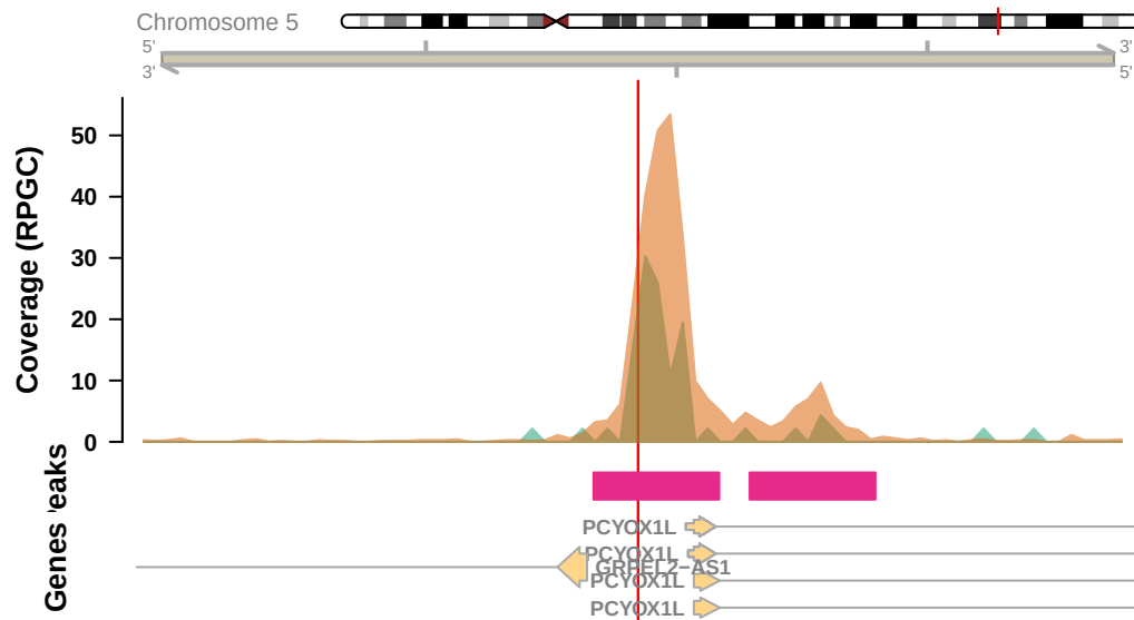
rs58729522 (PCYOX1L),Promoter (&lt;=1kb)
