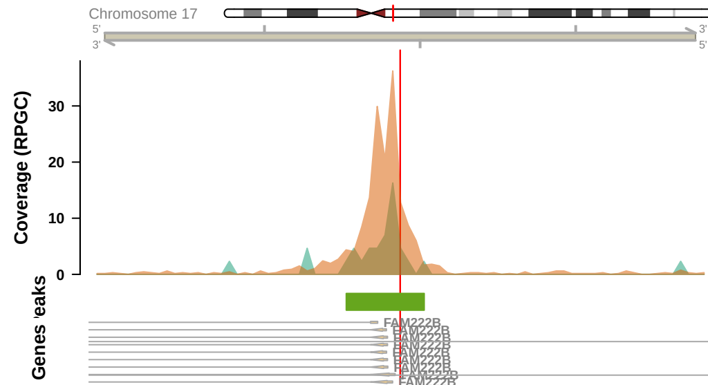
rs9890212 (FAM222B),Promoter (&lt;=1kb)
