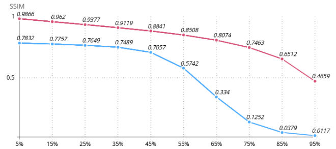
Abb. 9: SSIM-Werte für JQA (rot) im Vergleich zu Median M2 (blau), Quelle: [6]
