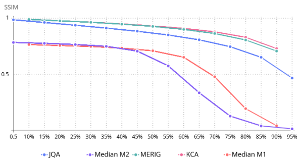
Abb. 11: SSIM-Werte aller Algorithmen im Vergleich zu Median M1 und M2, Quelle: [7] [20] [6] [5]
