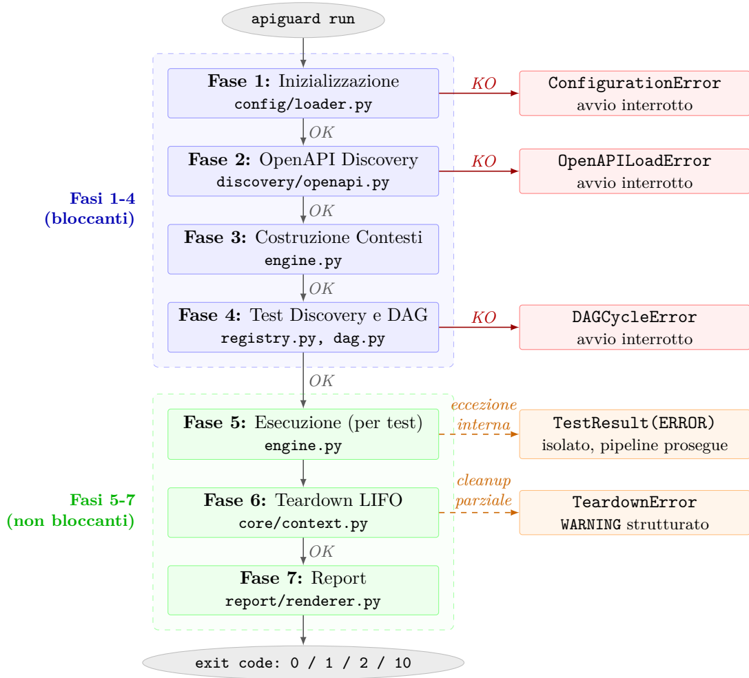
Figura 4.2: Pipeline a sette fasi: startup bloccante (Fasi 1–4) ed esecuzione non bloccante (Fasi 5–7).
