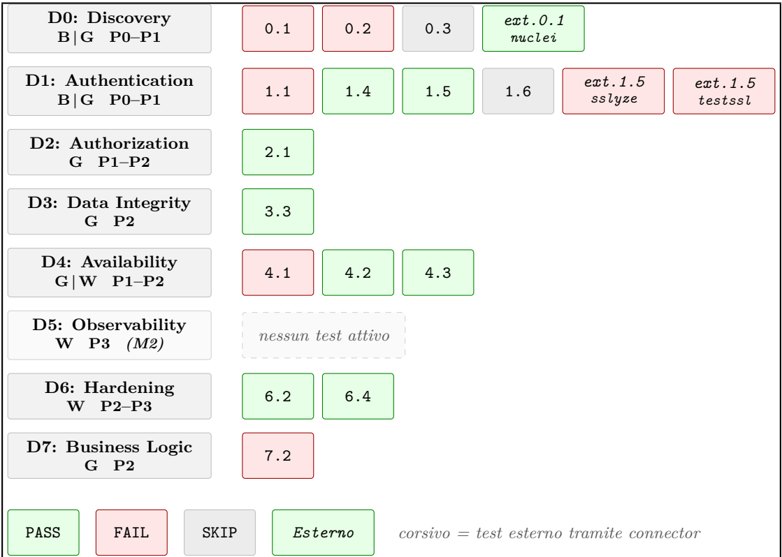
Figura 5.2: Mappa di copertura (v0.1.0): test attivi per dominio, strategia Box Gradient e esiti PASS/FAIL/SKIP.
