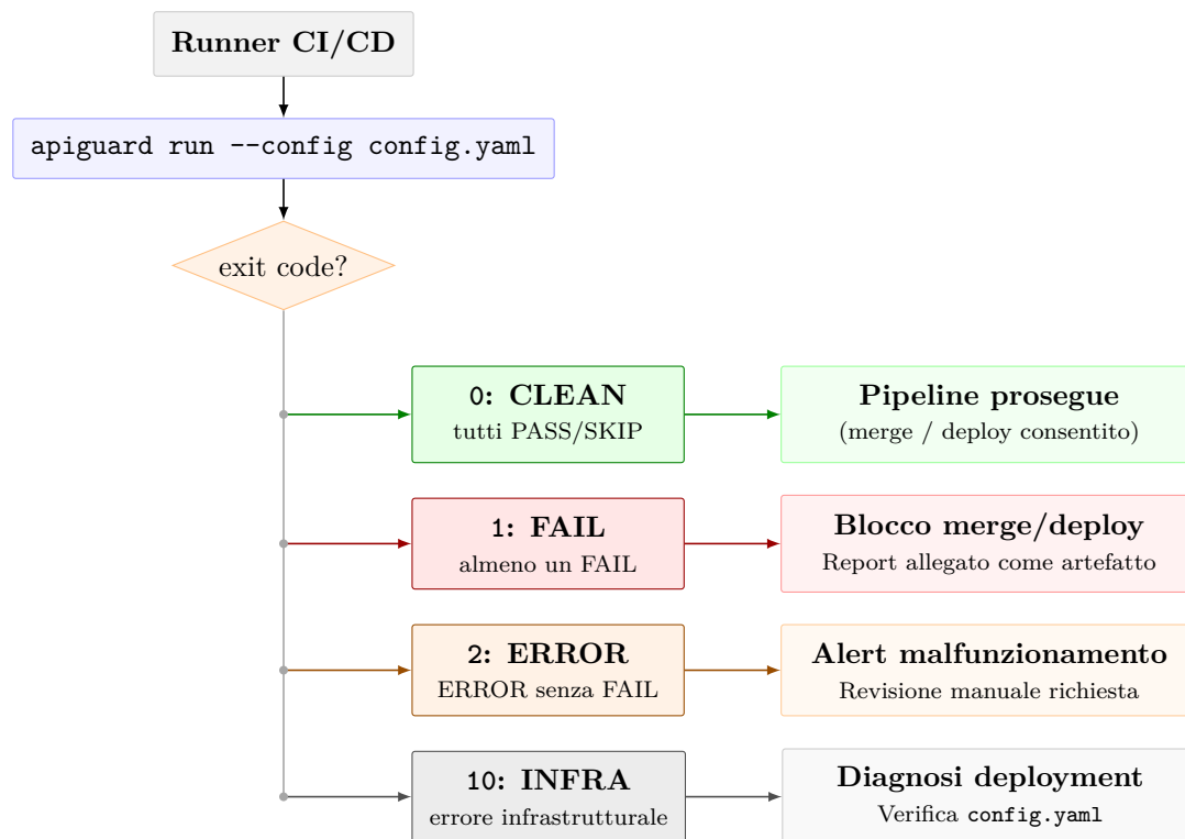
Figura 6.1: Routing degli exit code semantici (D6.P1) nella pipeline CI/CD: 0 clean, 1 fail, 2 error, 10 infra.
