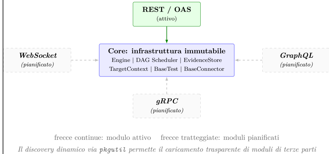
Figura 6.2: Evoluzione di APIGuard Assurance verso una piattaforma modulare: core immutabile e moduli di protocollo intercambiabili.
