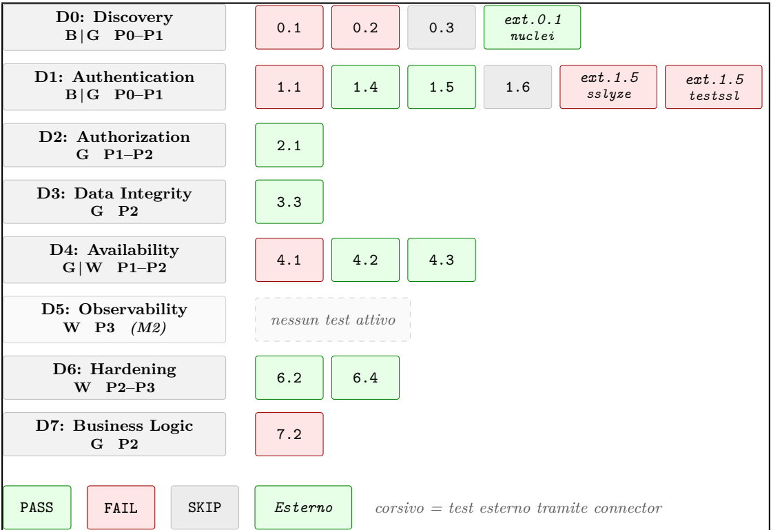
Figura 5.2: Mappa di copertura (v0.1.0): test attivi per dominio, strategia Box Gradient e esiti PASS/FAIL/SKIP.
