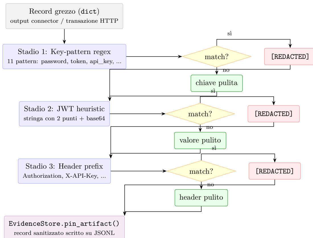
Figura 8.6: Sanitizzazione a imbuto dell'evidenza (D4.P2): key-pattern, JWT heuristic e header prefix in sequenza.
