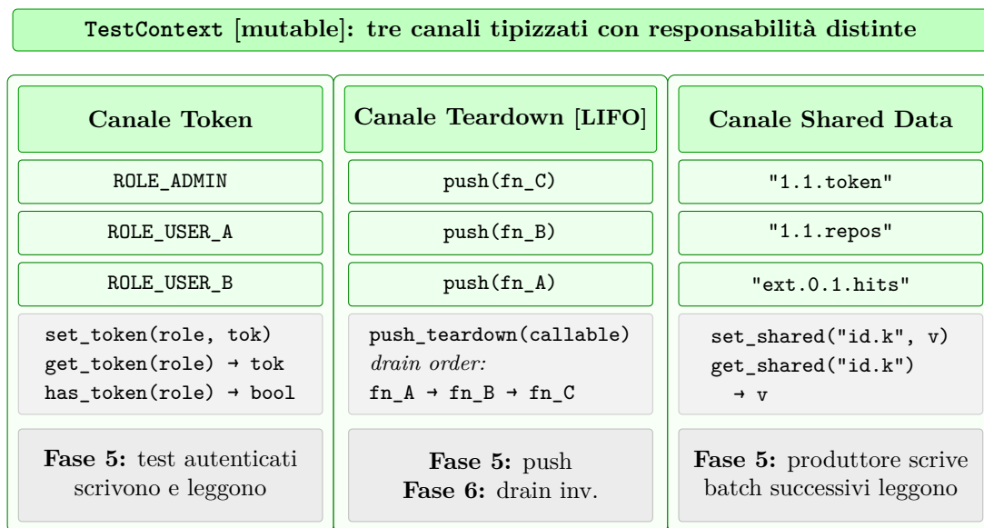
Figura 4.5: Struttura interna del TestContext (D1.P3): canali Token, Teardown LIFO e Shared Data.
