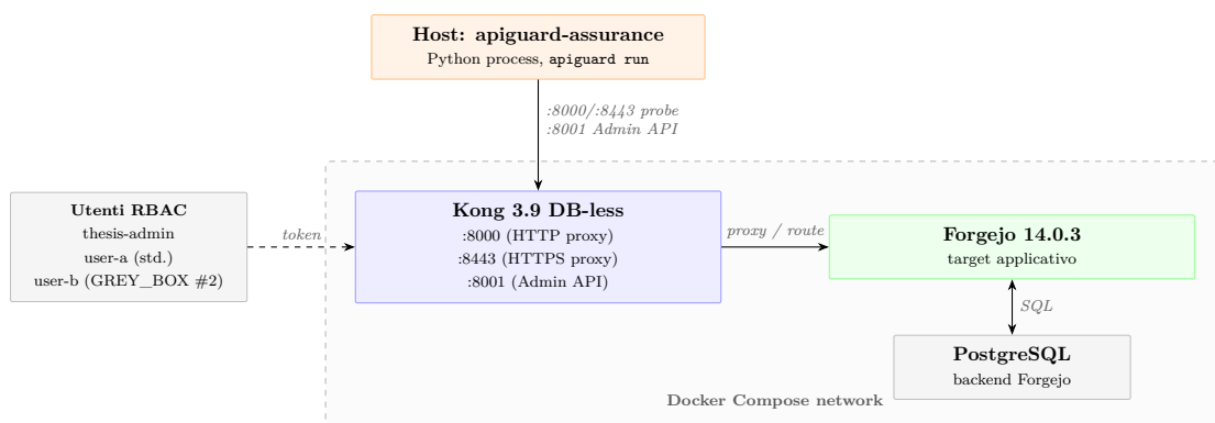
Figura 8.7: Topologia dell'ambiente di validazione sperimentale (Forgejo 14.0.3 + Kong 3.9 DB-less, Docker Compose).
