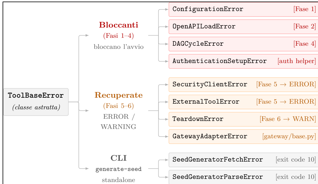
Figura 4.4: Gerarchia delle 11 eccezioni custom: bloccanti (Fasi 1-4), recuperate (Fasi 5-6) e CLI
