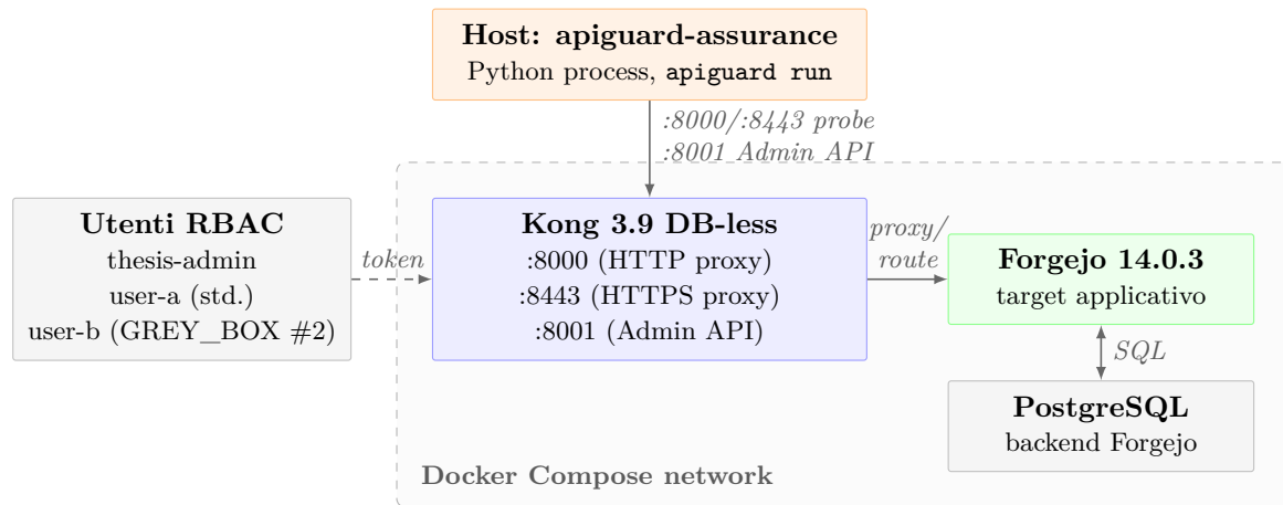
Figura 8.11: Topologia dell'ambiente di validazione sperimentale (Forgejo 14.0.3 + Kong 3.9 DB-less, Docker Compose).
