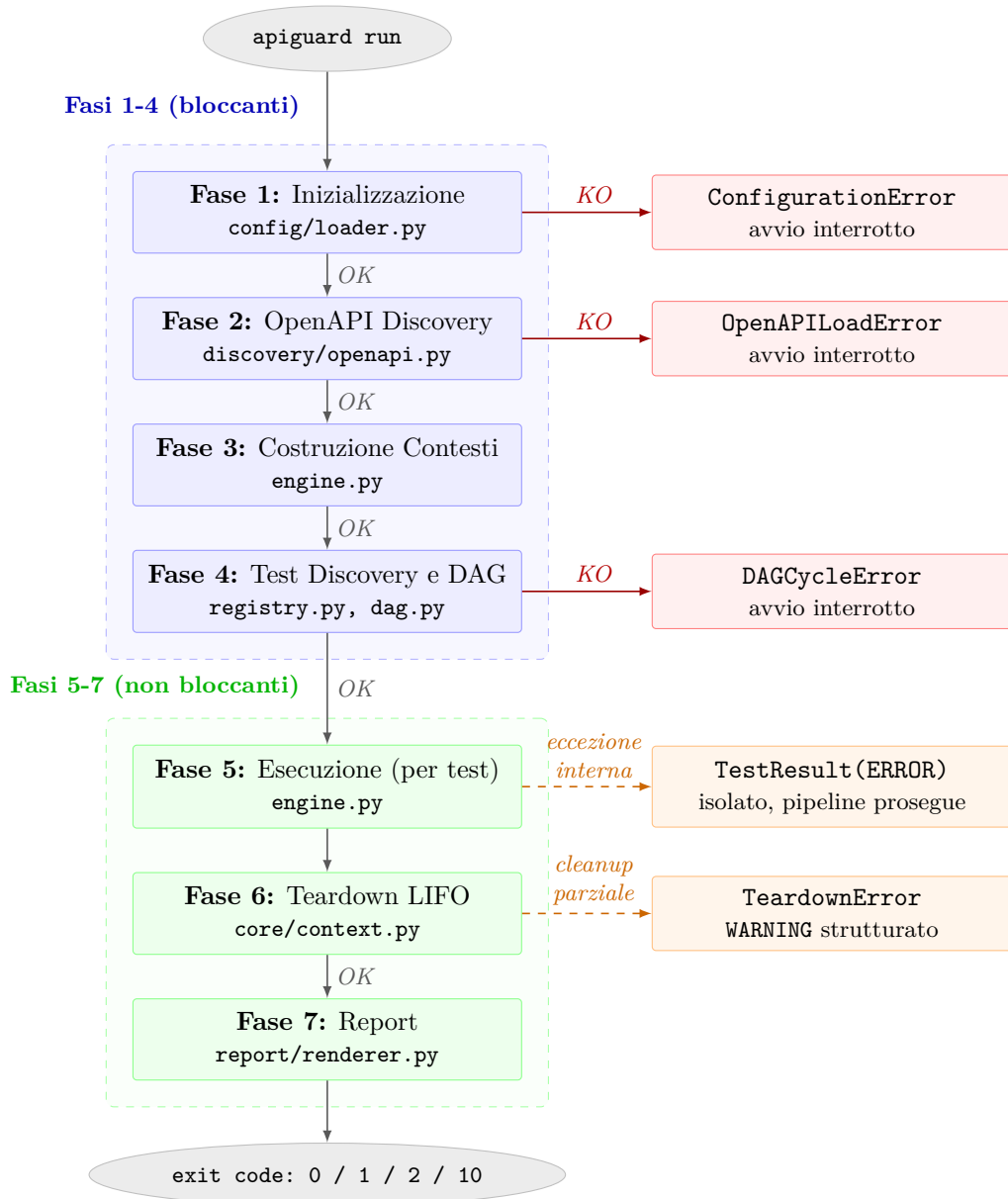
Figura 8.4: Flusso della pipeline a sette fasi (D4.P3, D4.P4): la zona di startup (Fasi 1-4) è bloccante, un errore in una qualsiasi di esse interrompe l'avvio; la zona di esecuzione (Fasi 5-7) è non bloccante, ogni malfunzionamento è recuperato localmente senza invalidare i risultati già prodotti. Freccie continue: percorso nominale; frecce tratteggiate: errori recuperati con WARNING .
