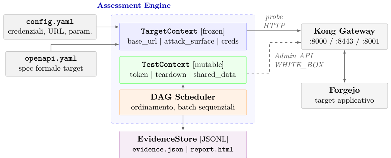
Figura 8.2: Architettura di alto livello di APIGuard Assurance: input, Engine con Split State (D1.P3), DAG Scheduler (D2.P2) ed EvidenceStore (D4.P1).
