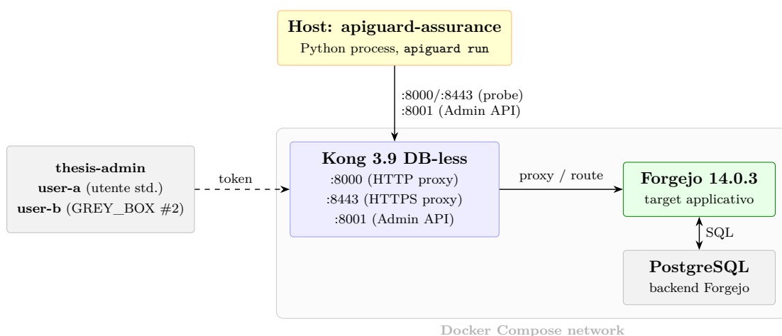
Figura 8.7: Topologia dell'ambiente di validazione sperimentale (Forgejo 14.0.3 + Kong 3.9 DB-less, Docker Compose).
