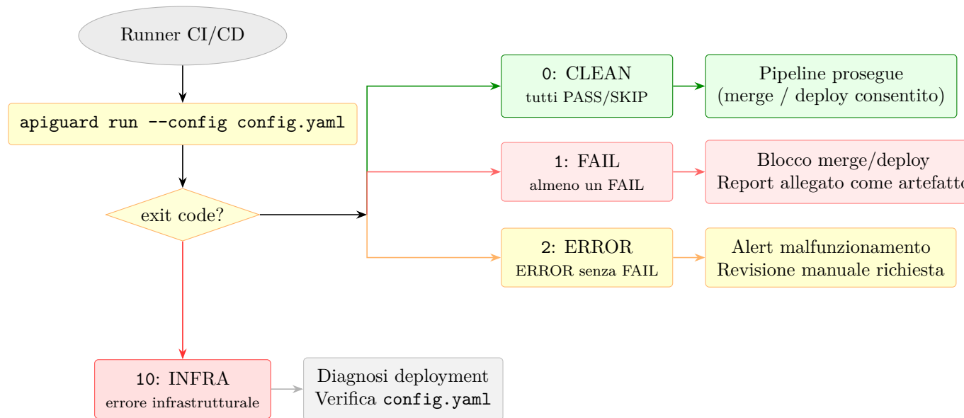
Figura 8.9: Routing degli exit code semantici (D6.P1) nella pipeline CI/CD: 0 clean, 1 fail, 2 error, 10 infra.
