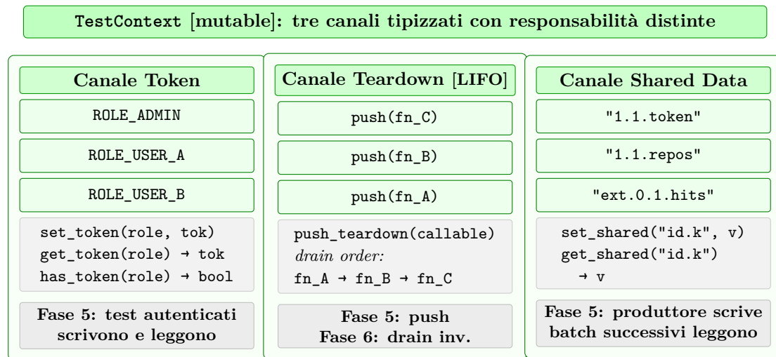
Figura 8.12: Struttura interna del TestContext (D1.P3): i tre canali tipizzati con le rispettive API di accesso, le chiavi costanti per il canale token, il pattern di naming per il canale shared e l'ordinamento LIFO del canale teardown.
