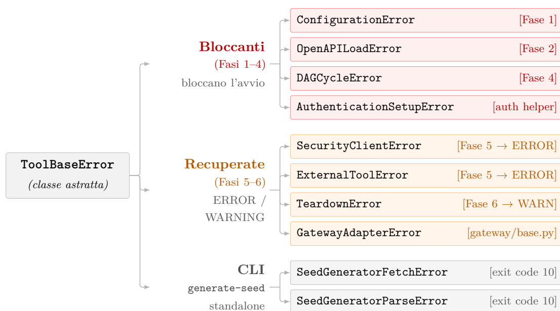
Figura 8.13: Gerarchia delle 11 eccezioni custom di APIGuard Assurance (D4.P4): eccezioni bloccanti che interrompono lo startup (Fasi 1-4, rosso), eccezioni recuperate localmente che producono TestResult(ERROR/WARNING) (Fasi 5-6, oro), e classi specifiche del comando CLI generate-seed (grigio). Tutte ereditano da ToolBaseError .
