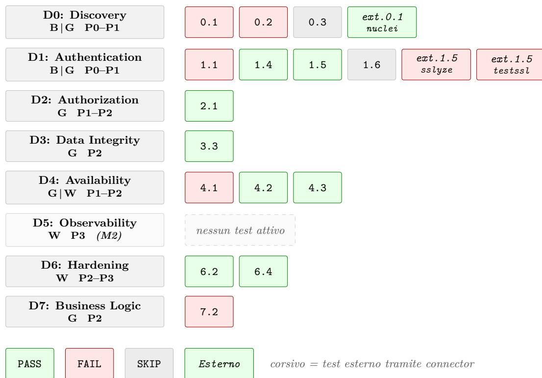
Figura 8.11: Mappa di copertura dell'assessment di validazione (v0.1.0): test attivi per dominio di assurance, strategia Box Gradient (D3.P3) ed esito (PASS/FAIL/SKIP). I test esterni, eseguiti tramite connector, sono riportati in corsivo.
