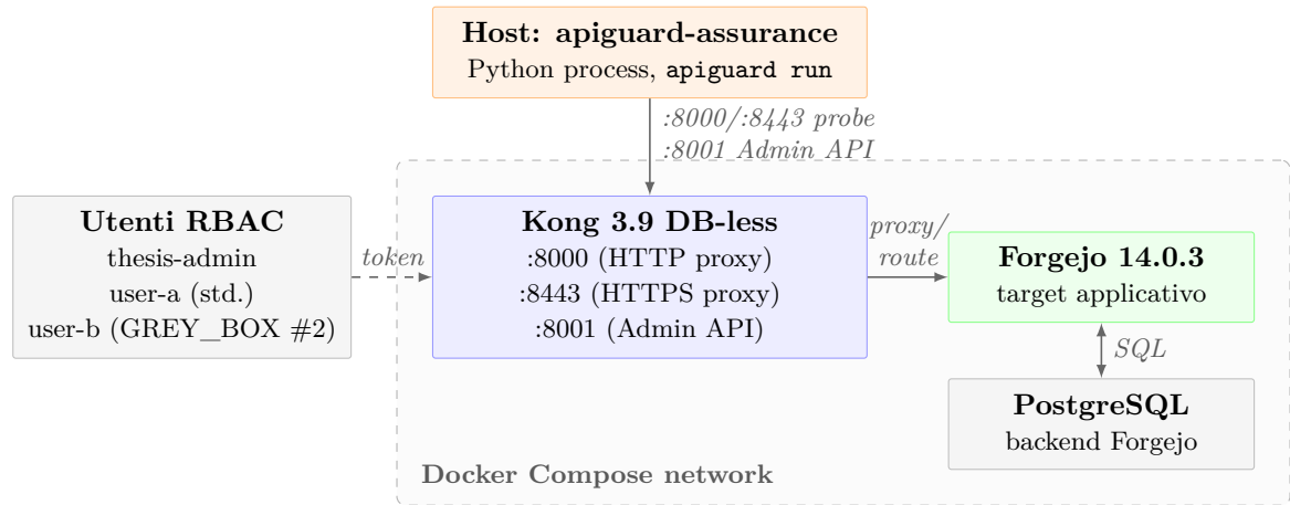
Figura 5.1: Topologia dell'ambiente di validazione sperimentale (Forgejo 14.0.3 + Kong 3.9 DB-less, Docker Compose).
