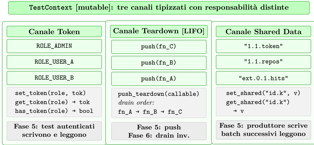
Figura 4.5: Struttura interna del TestContext (D1.P3): canali Token, Teardown LIFO e Shared Data.
