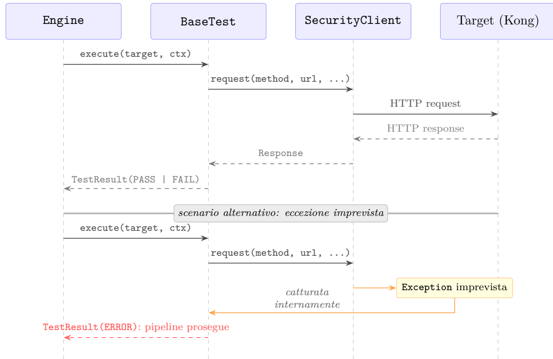
Figura 4.3: Ciclo di vita di un test in Fase 5: scenario normale e scenario di eccezione con error isolation (D4.P3).
