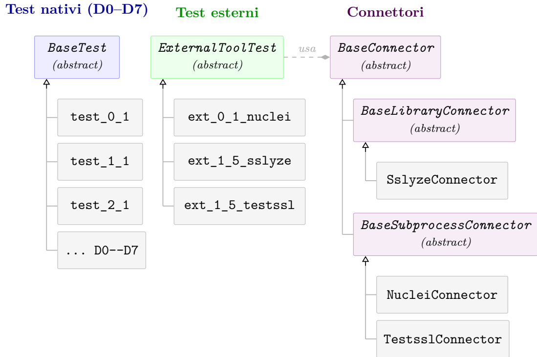
Figura 4.7: Gerarchia duale BaseTest / ExternalToolTest (D1.P4) e gerarchia dei connettori Library / Subprocess (D1.P5).
