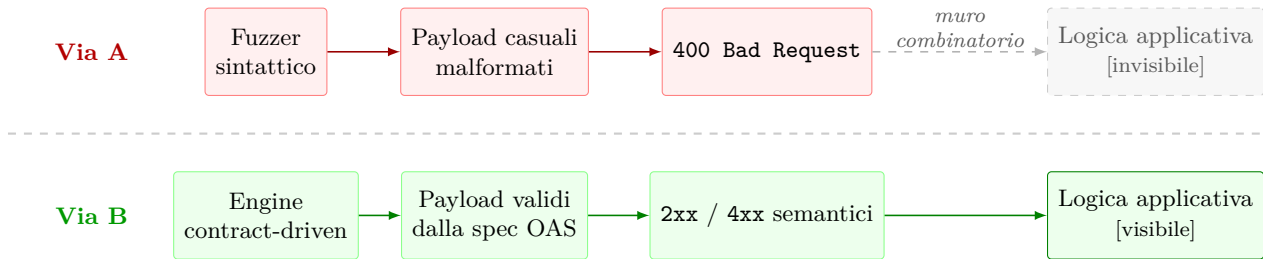
Figura 2.1: Il combinatorial wall : fuzzer sintattico (Via A) vs. approccio contract-driven OAS (Via B).
