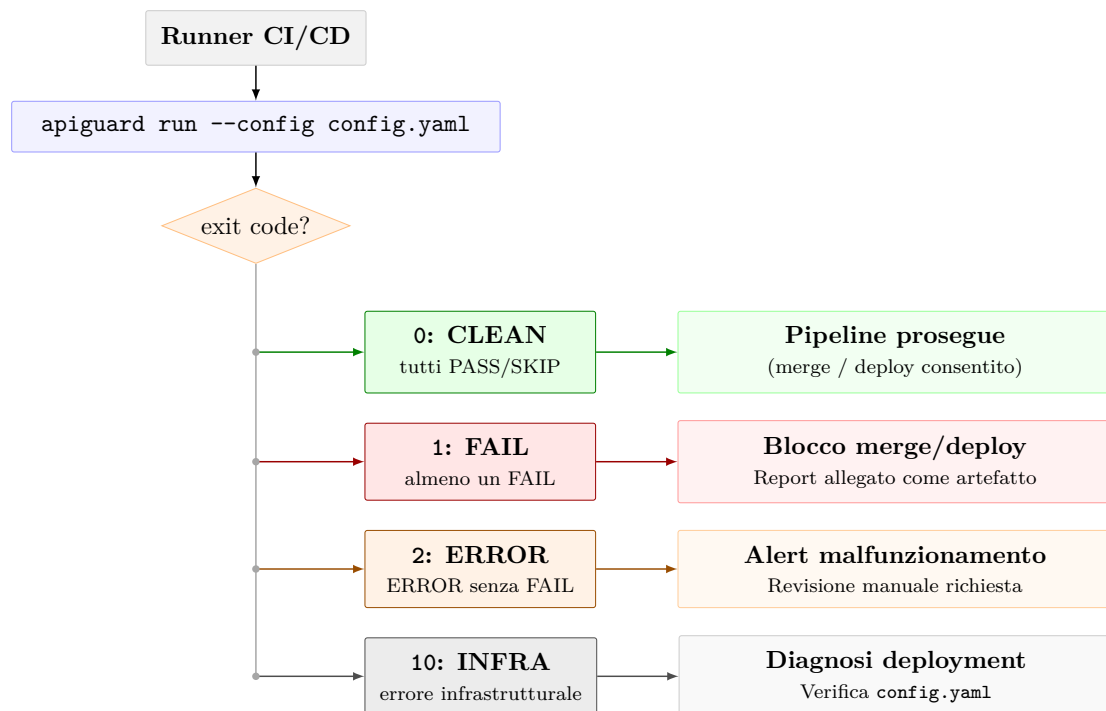
Figura 6.1: Routing degli exit code semantici (D6.P1) nella pipeline CI/CD: 0 clean, 1 fail, 2 error, 10 infra.
