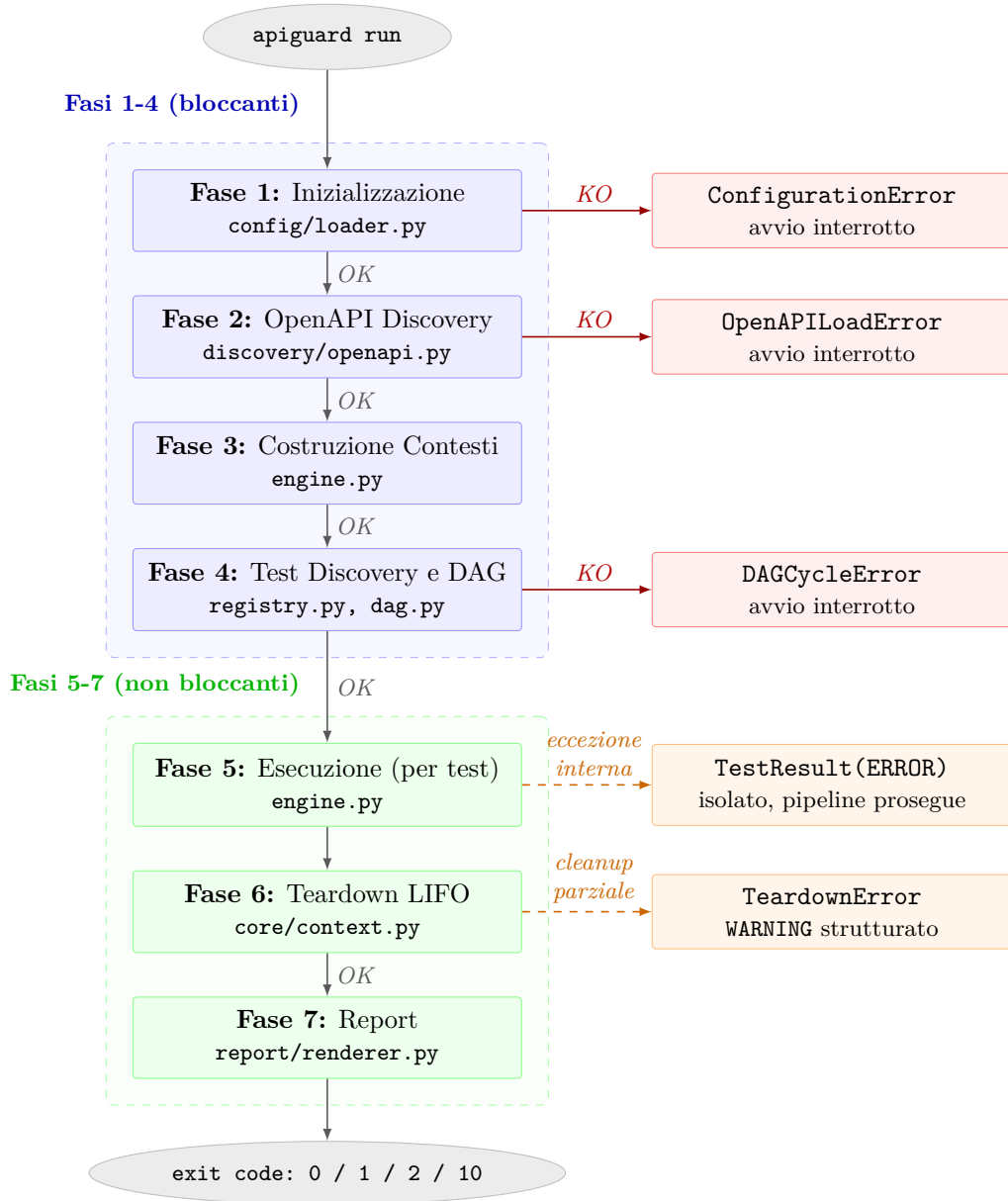
Figura 4.2: Pipeline a sette fasi: startup bloccante (Fasi 1–4) ed esecuzione non bloccante (Fasi 5–7).
