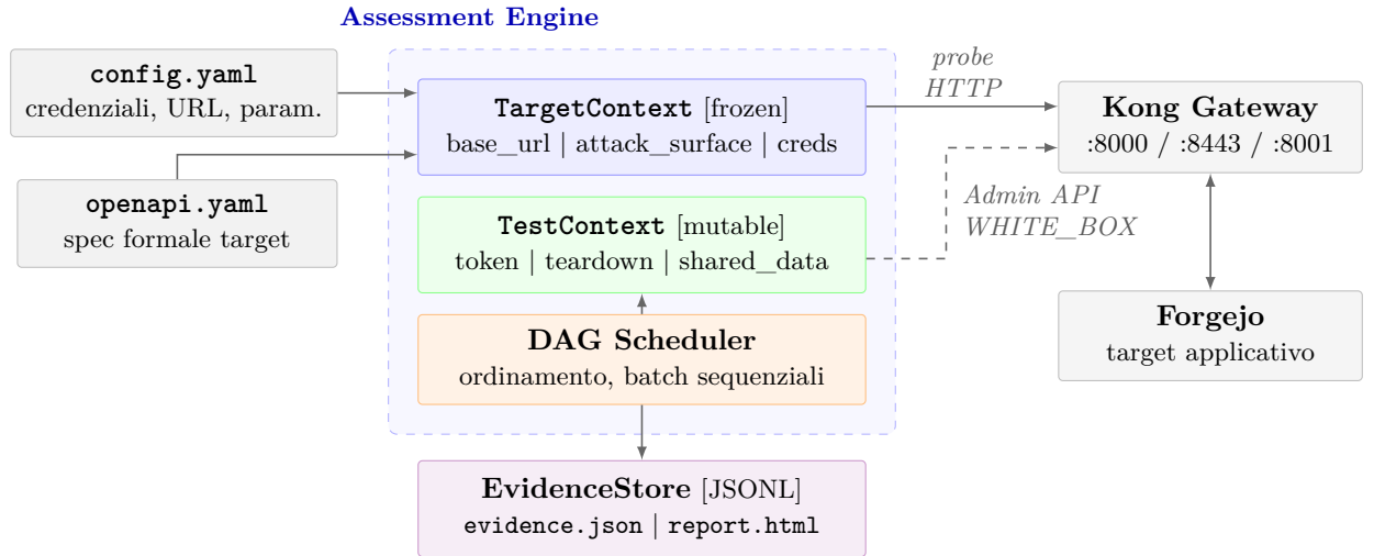
Figura 3.1: Architettura di APIGuard Assurance: Engine, DAG Scheduler ed Evidence-Store.
