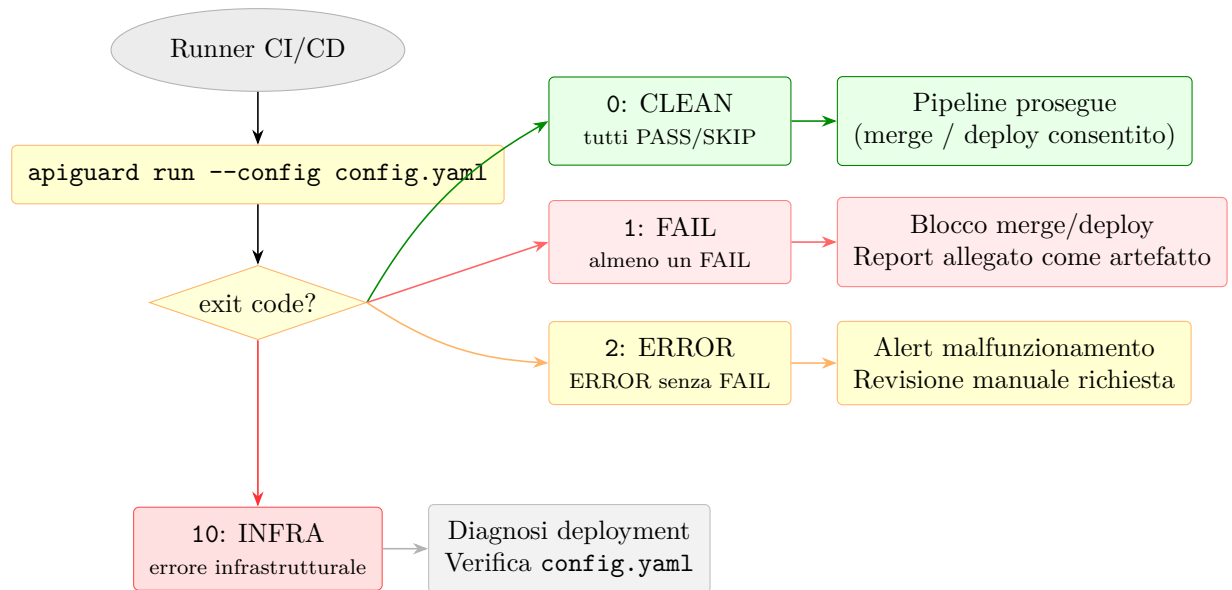
Figura 7.9: Routing degli exit code semantici (D6.P1) nella pipeline CI/CD: 0 clean, 1 fail, 2 error, 10 infra.
