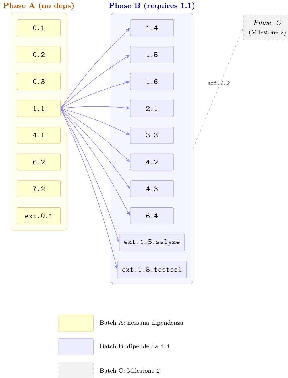
Figura 7.3: Topologia del DAG di dipendenza in Milestone 1: Phase A (no deps), Phase B (requires 1.1) e Phase C pianificata (Milestone 2).
