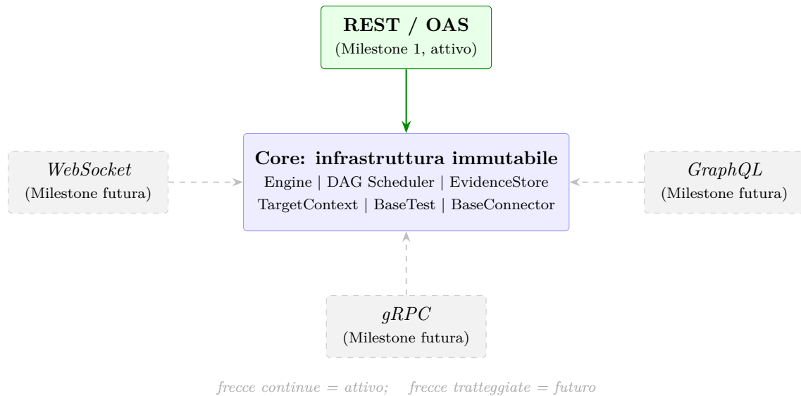
Figura 7.10: Evoluzione di APIGuard Assurance verso una piattaforma modulare: core immutabile e moduli di protocollo intercambiabili.
