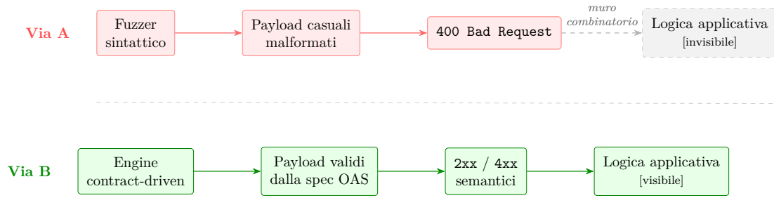
Figura 7.1: Il combinatorial wall : fuzzer sintattico (Via A) vs. approccio contract-driven OAS (Via B).
