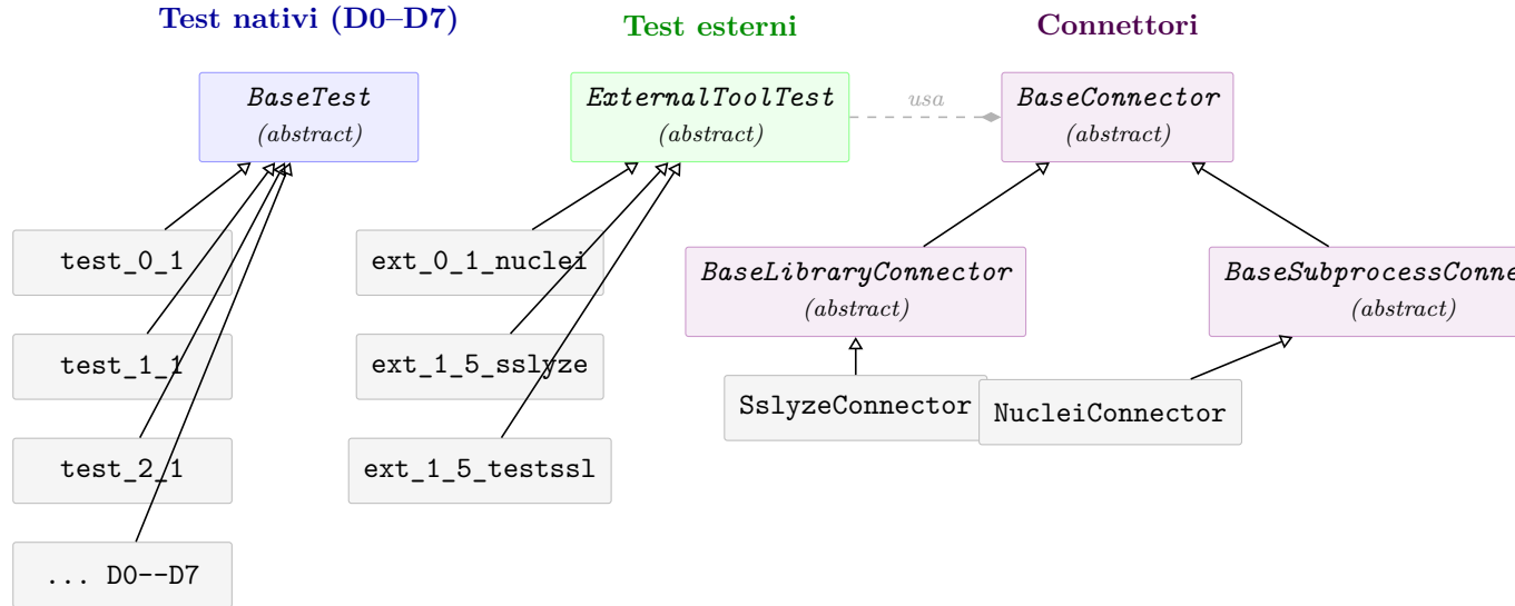
Figura 7.5: Gerarchia duale BaseTest / ExternalToolTest (D1.P4) e gerarchia dei connettori Library / Subprocess (D1.P5).
