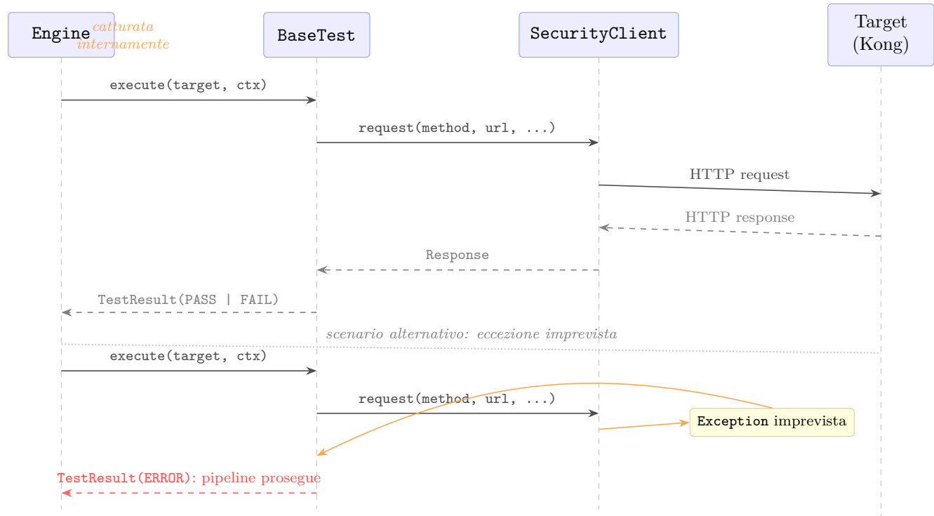
Figura 7.4: Ciclo di vita di un test in Fase 5: scenario normale e scenario di eccezione con error isolation (D4.P3).
