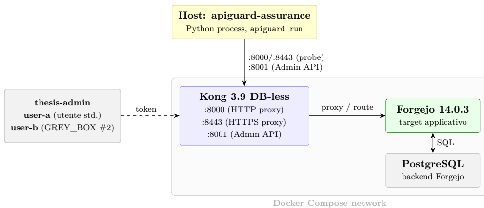
Figura 7.7: Topologia dell'ambiente di validazione sperimentale (Forgejo 14.0.3 + Kong 3.9 DB-less, Docker Compose).
