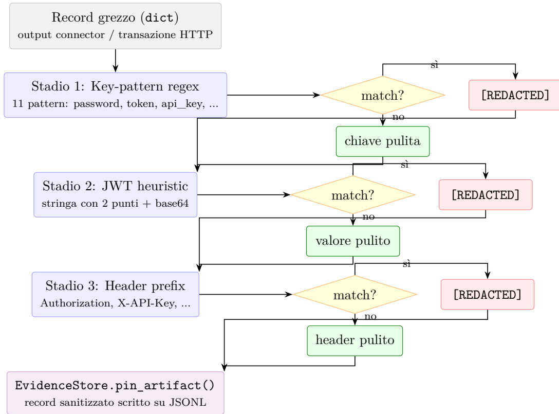
Figura 7.6: Sanitizzazione a imbuto dell'evidenza (D4.P2): key-pattern, JWT heuristic e header prefix in sequenza.
