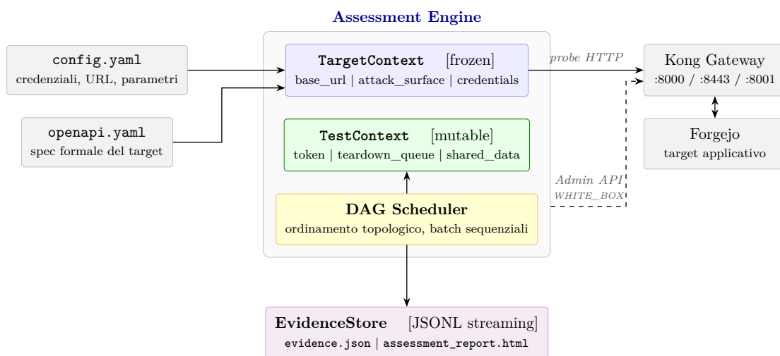
Figura 8.2: Architettura di alto livello di APIGuard Assurance: input, Engine con Split State (D1.P3), DAG Scheduler (D2.P2) ed EvidenceStore (D4.P1).
