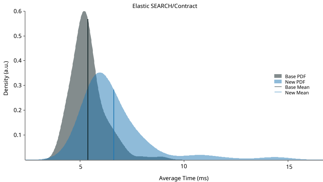
Figura 5.1: Diagramma confronto densità probabilistica richieste evaluate di tipo SEARCH
