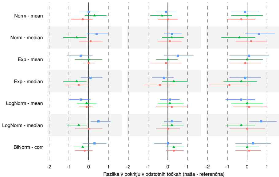
Enostranski spodnji interval
