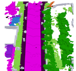
G.T. Occupancy
