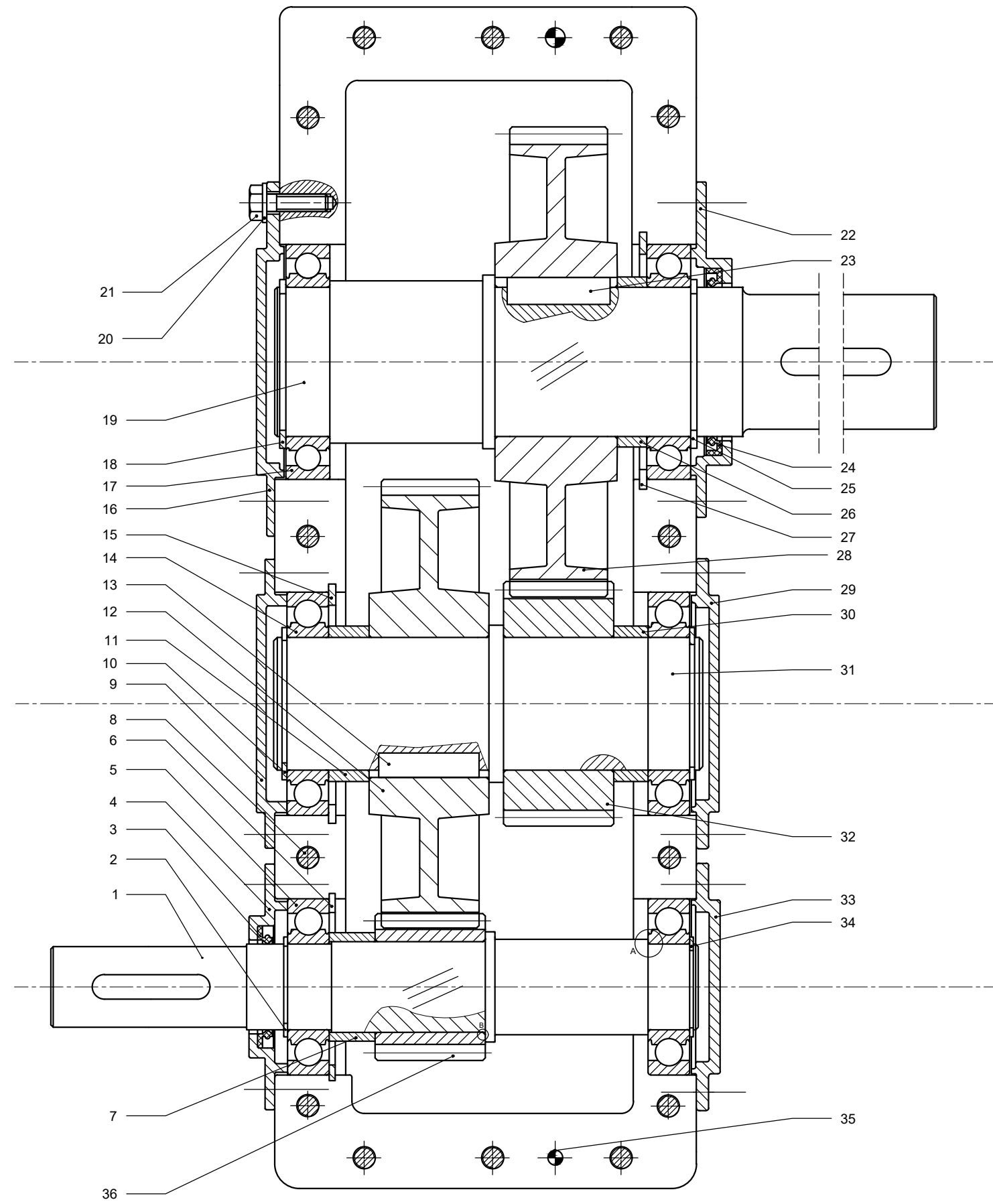
DETAY A
