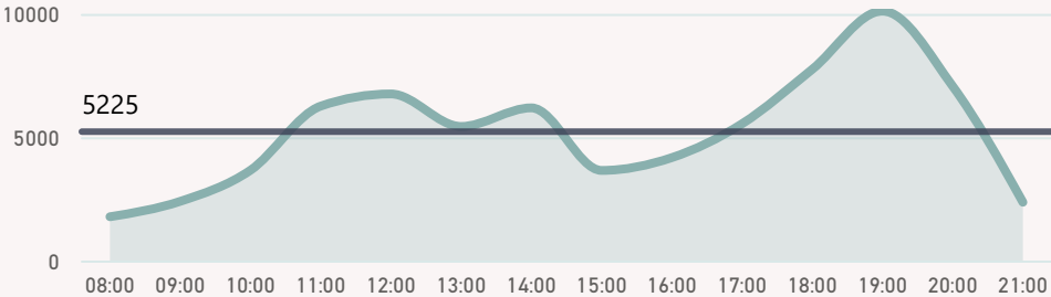
Qtde de Pedidos por Hora
