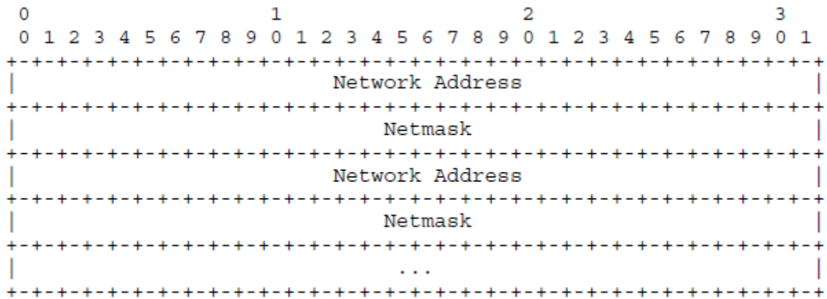
Figure A. 3:HNA Message fields
