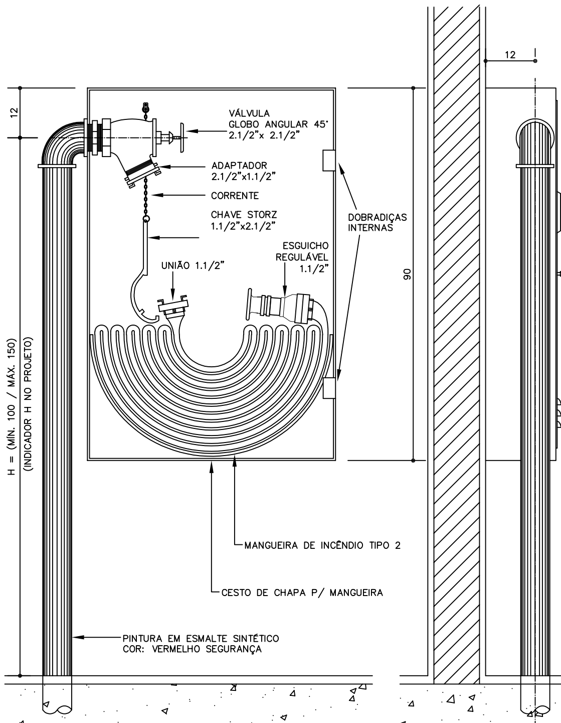
VISTA FRONTAL (INTERNA) ESC. 1:10
