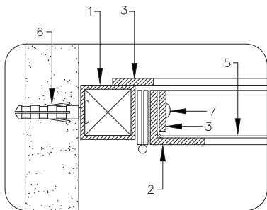
DETALHE 1 ESCALA 1:2,5
