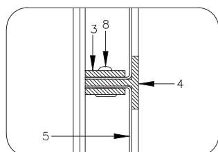
DETALHE 4 ESCALA 1:2,5
