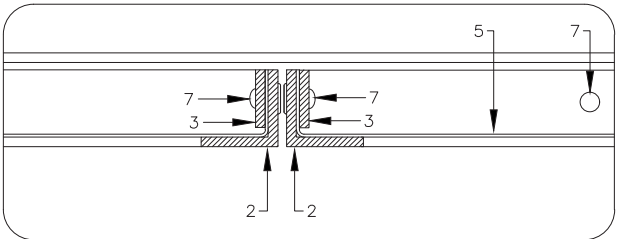
DETALHE 2 ESCALA 1:2,5
