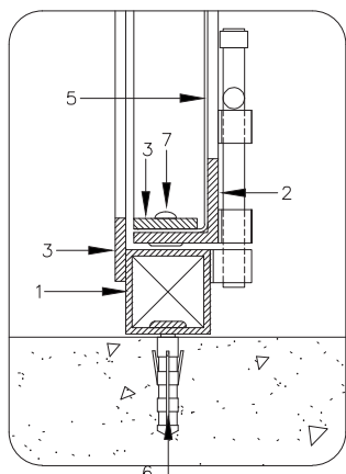
DETALHE 5 ESCALA 1:2,5
