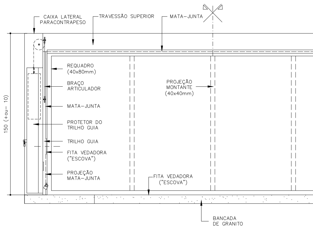
AMPLIAÇÃO PARCIAL – VISTA INTERNA ESCALA 1:20
