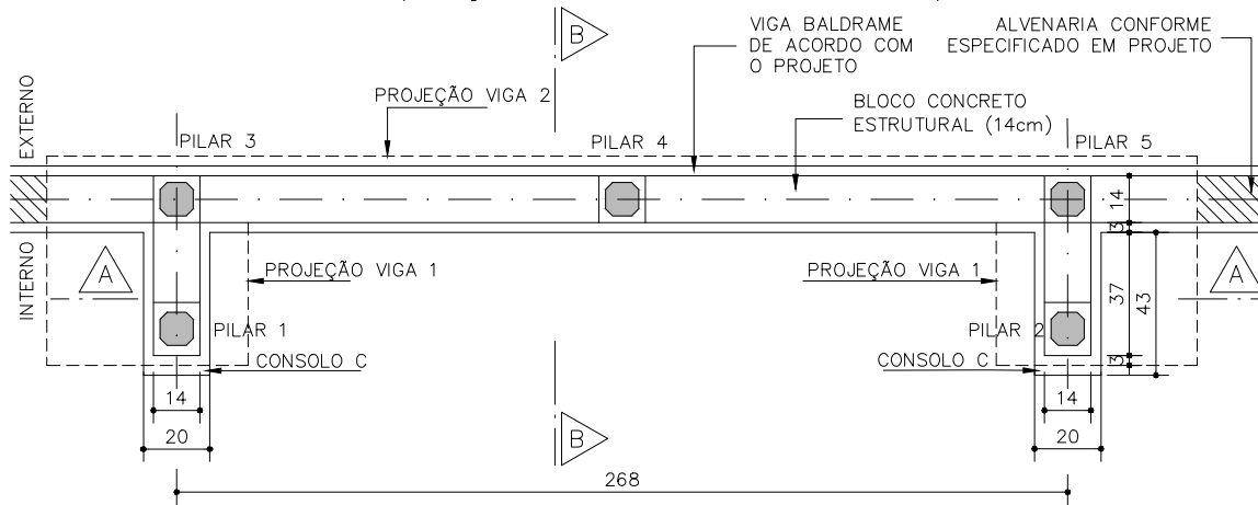
PLANTA ESCALA 1:25
