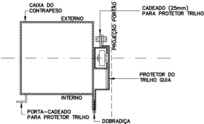
DETALHE PROTETOR DO TRILHO-GUIA (POSIÇÃO PORTA ABERTA) ESCALA 1:5
