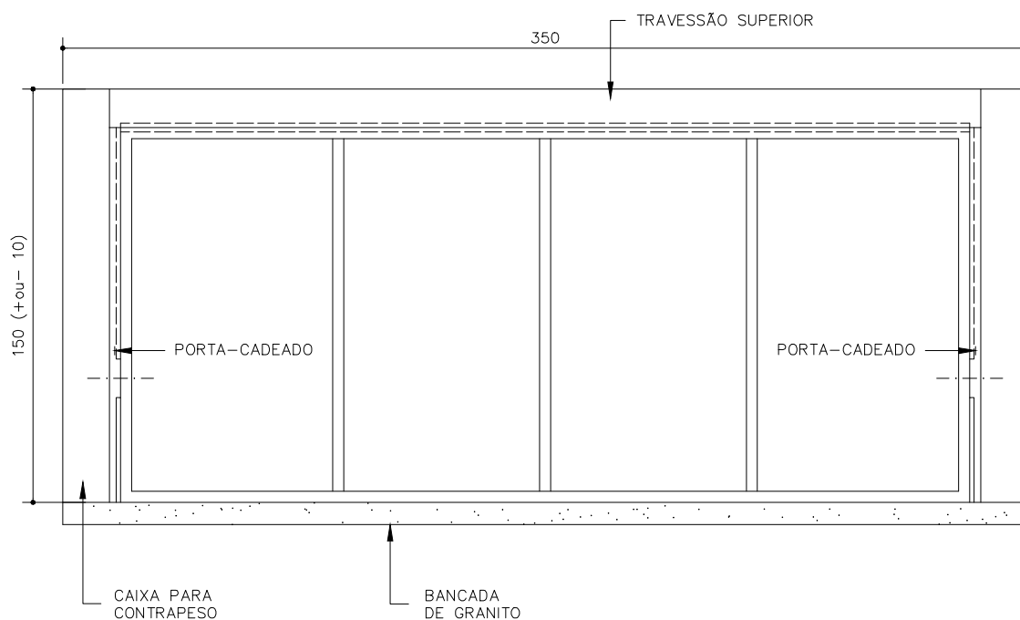
VISTA 2 ESCALA 1:25
