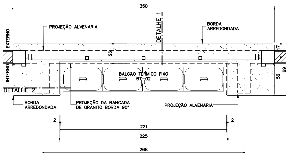
PLANTA BA-10 COM BT-02
