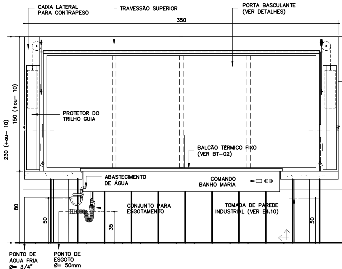
VISTA 1
