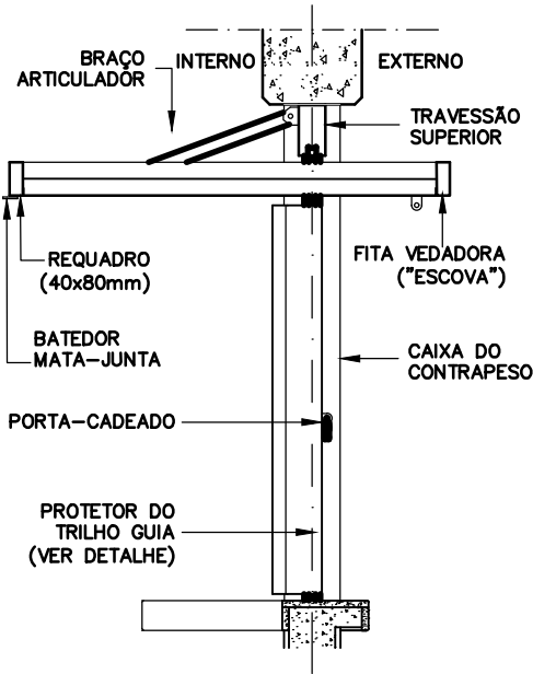
CORTE CC POSIÇÃO ABERTA ESCALA 1:25
