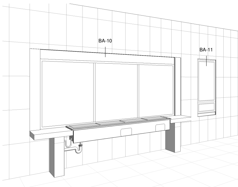
EXEMPLO DE COMPOSIÇÃO BA-10 E BA-11 - VISTA INTERNA
