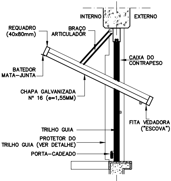
CORTE DD POSIÇÃO SEMI-ABERTA ESCALA 1:25
