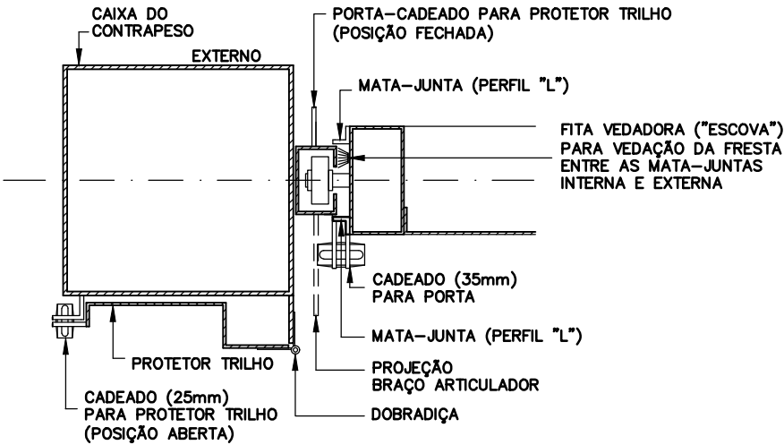
DETALHE PROTETOR DO TRILHO-GUIA (POSIÇÃO PORTA FECHADA)
