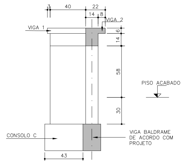
CORTE BB ESCALA 1:25
