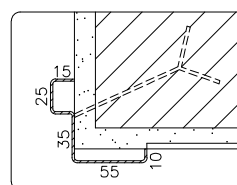
DETALHE BATENTE ESCALA 1:5 (MEDIDAS EM mm)
