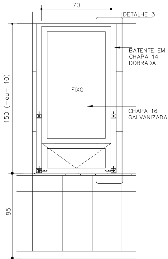
VISTA 2 INTERNA ESCALA 1:25
