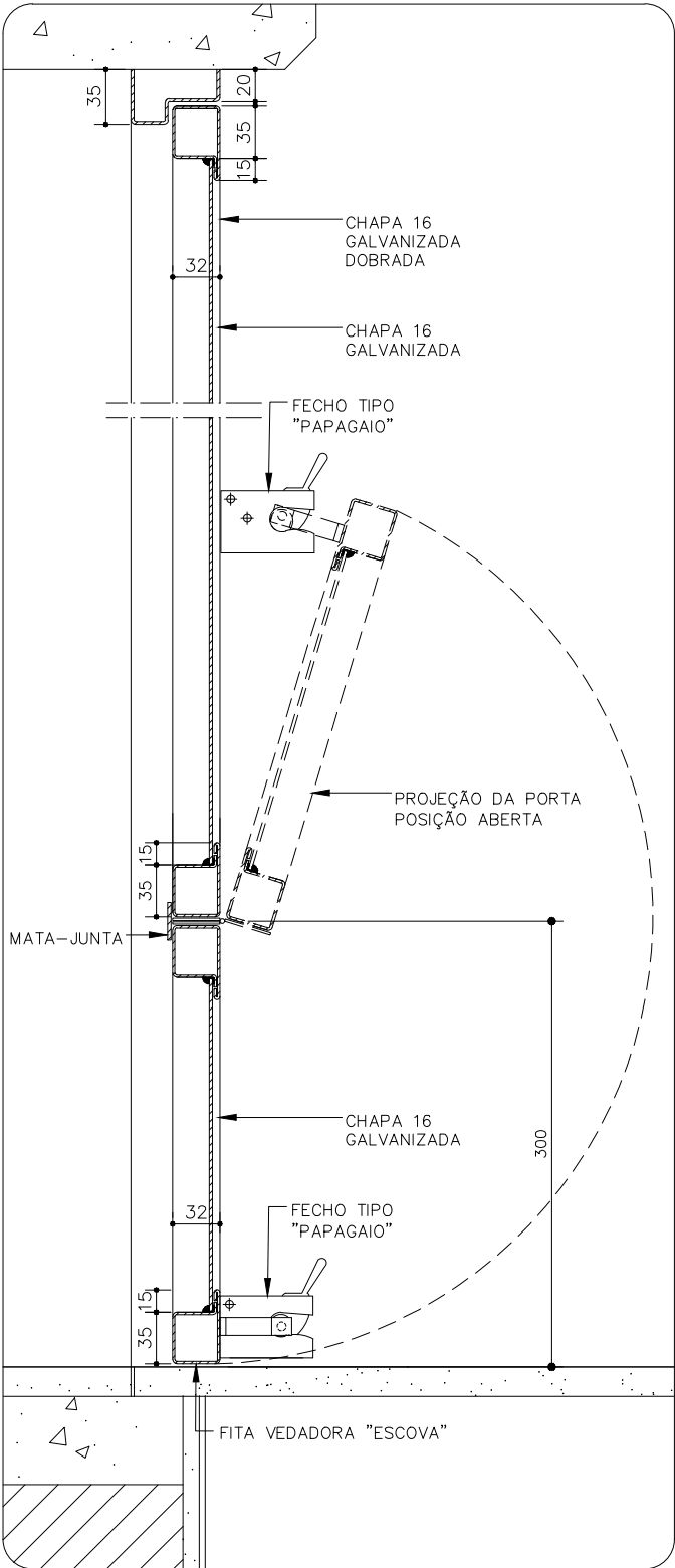
DETALHE 4 ESCALA 1:5
