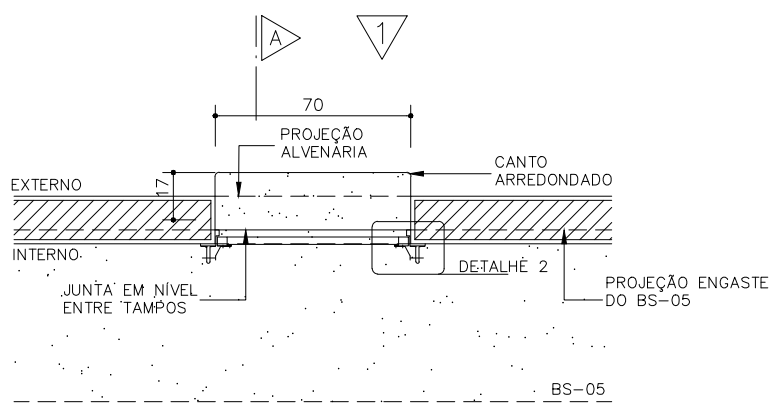
PLANTA ESCALA 1:25
