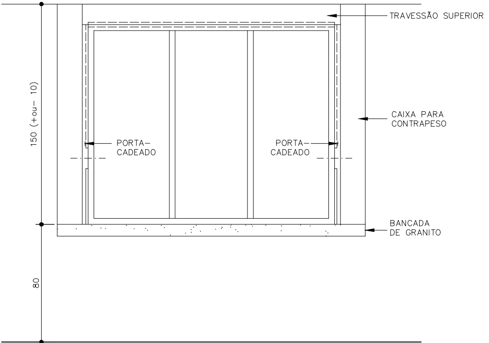
VISTA 1 ESCALA 1:25
