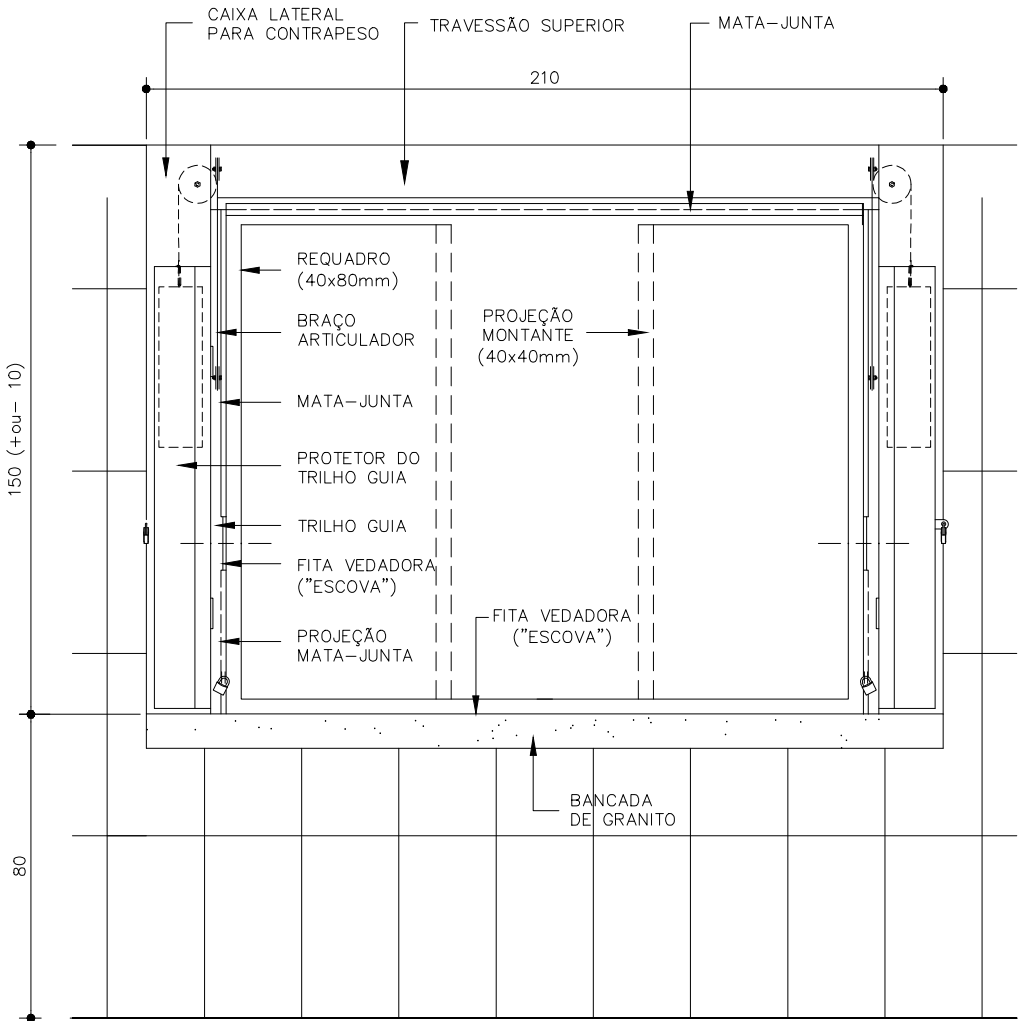
VISTA 2 – PORTA BASCULANTE ESCALA 1: 20
