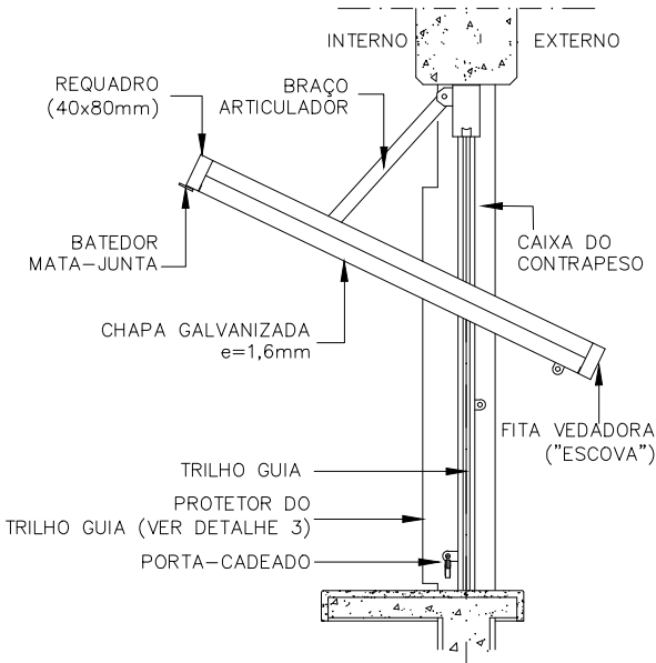
CORTE CC POSIÇÃO SEMI-ABERTA ESCALA 1: 25
