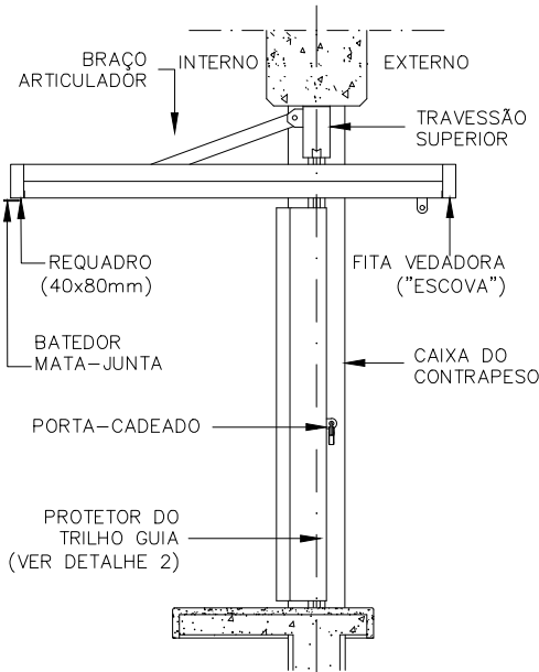
CORTE BB POSIÇÃO ABERTA ESCALA 1: 25
