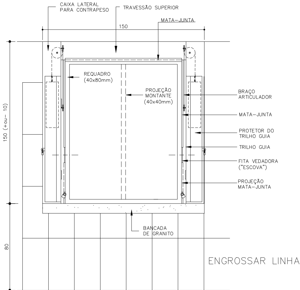
VISTA 2 – PORTA BASCULANTE ESCALA 1:20
