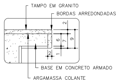
DETALHE 1 ESCALA 1:10
