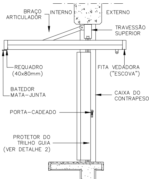
CORTE BB POSIÇÃO ABERTA ESCALA 1:25
