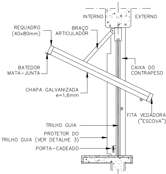
CORTE CC POSIÇÃO SEMI-ABERTA ESCALA 1:25
