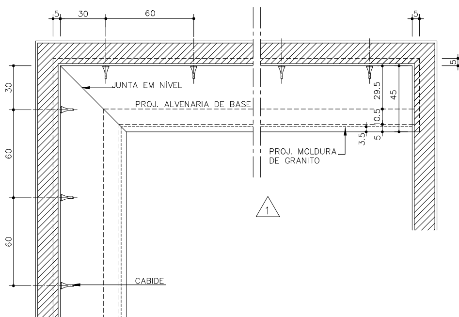
PLANTA ESC. 1:25
