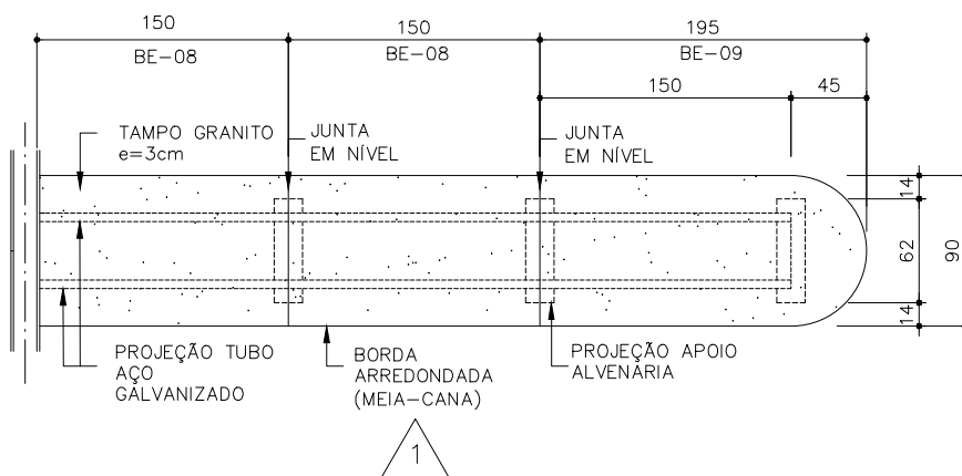
PLANTA TAMPO DA BANCADA ESCALA 1:50
