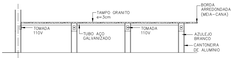
VISTA 1 ESCALA 1:50
