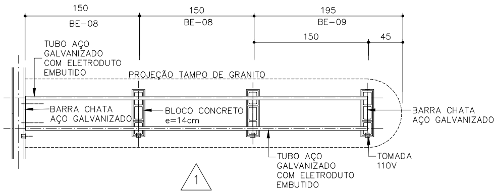
PLANTA BASE DE APOIOS ESCALA 1:50
