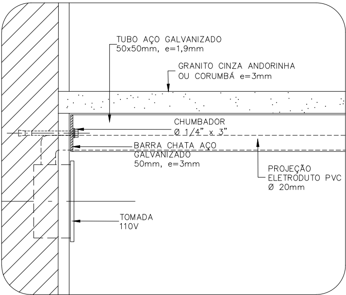
DETALHE 1 ESCALA 1:5
