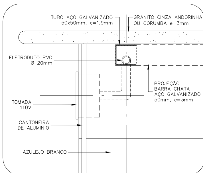
DETALHE 3 ESCALA 1:5
