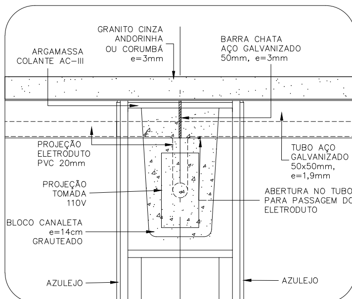
DETALHE 2 ESCALA 1:5
