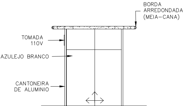
VISTA 2 ESCALA 1:25
