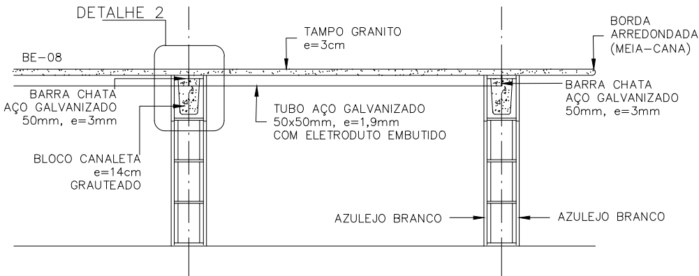
CORTE LONGITUDINAL ESCALA 1:25
