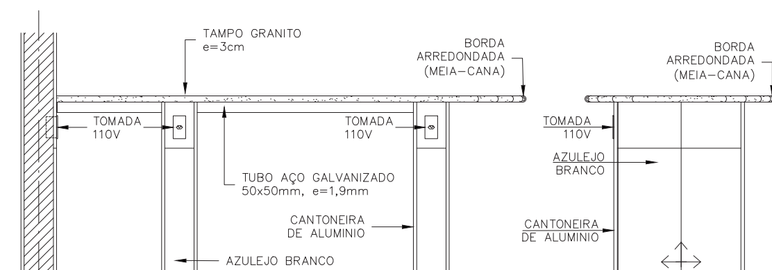
VISTA 1 ESCALA 1:25
