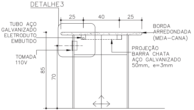
CORTE BB ESCALA 1:25
