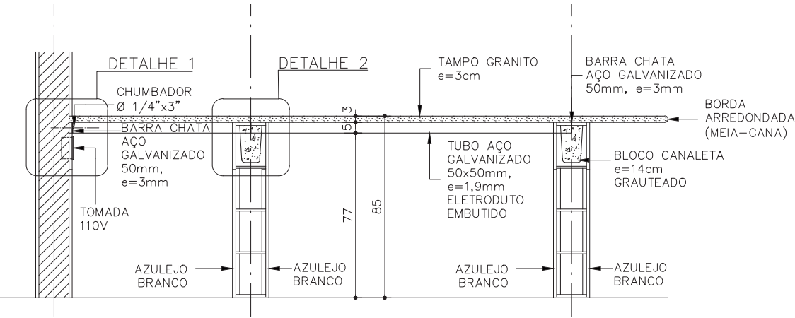
CORTE LONGITUDINAL ESCALA 1:25
