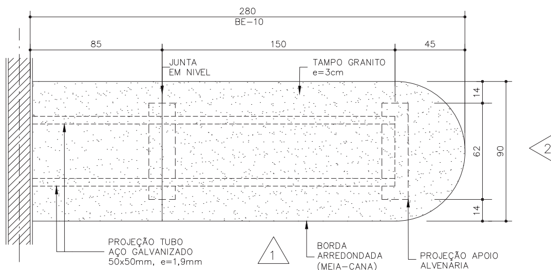
PLANTA TAMPO DA BANCADA ESCALA 1:25
