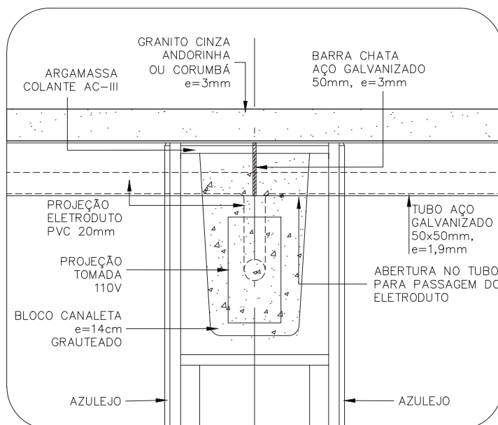
DETALHE 2 ESCALA 1:5
