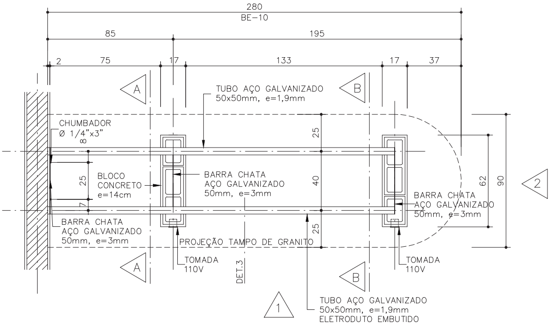
PLANTA BASE DE APOIOS ESCALA 1:25
