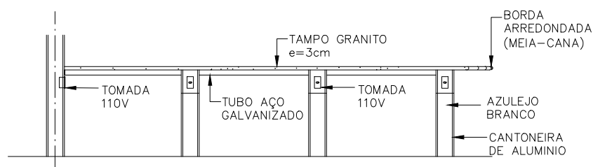
VISTA 1 ESCALA 1:50
