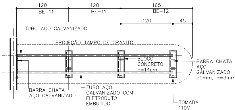
PLANTA BASE DE APOIOS ESCALA 1:50
