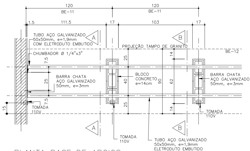
PLANTA BASE DE APOIOS ESCALA 1:25
