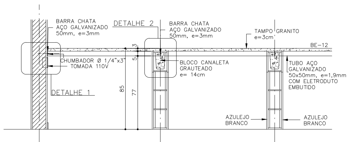
CORTE LONGITUDINAL ESCALA 1:25
