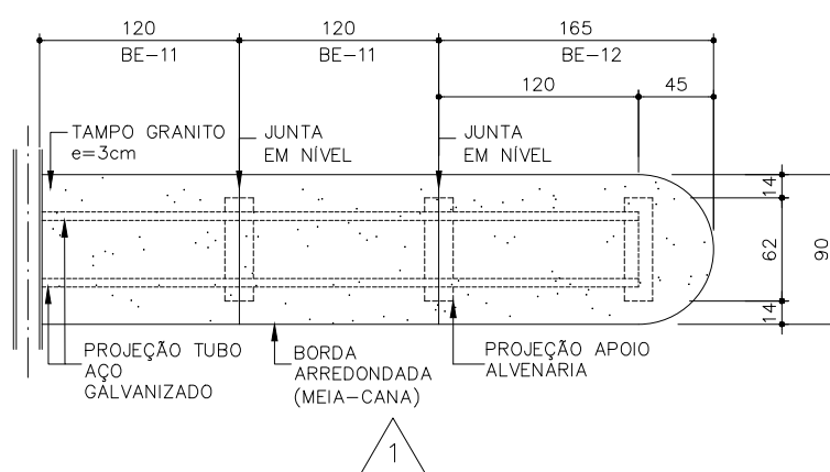
PLANTA TAMPO DA BANCADA ESCALA 1:50
