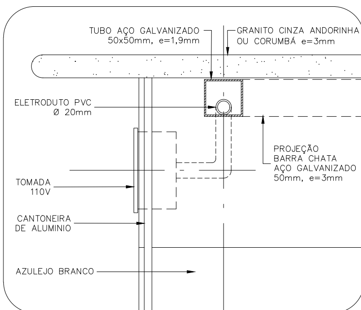
DETALHE 3 ESCALA 1:5
