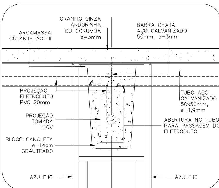
DETALHE 2 ESCALA 1:5
