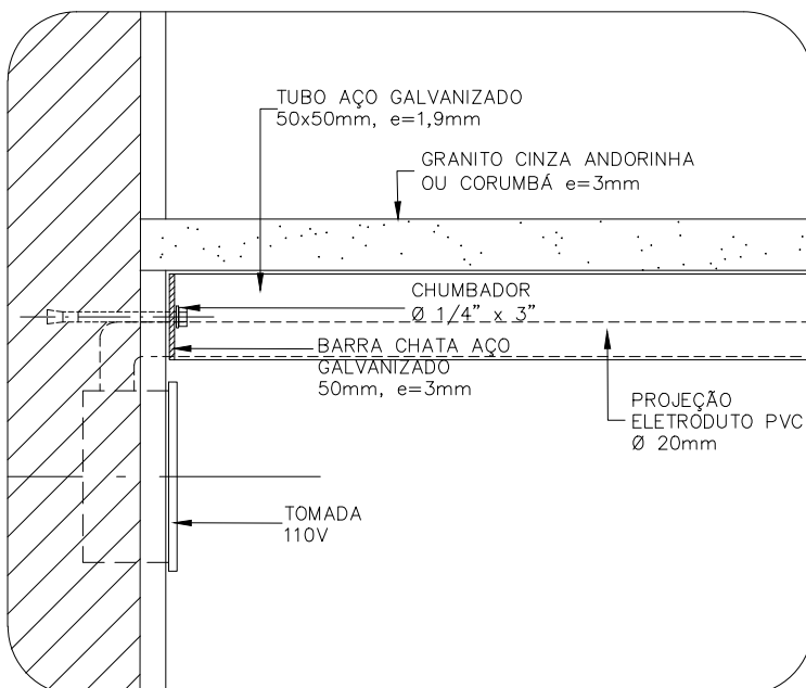
DETALHE 1 ESCALA 1:5
