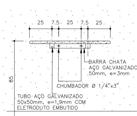
CORTE AA
