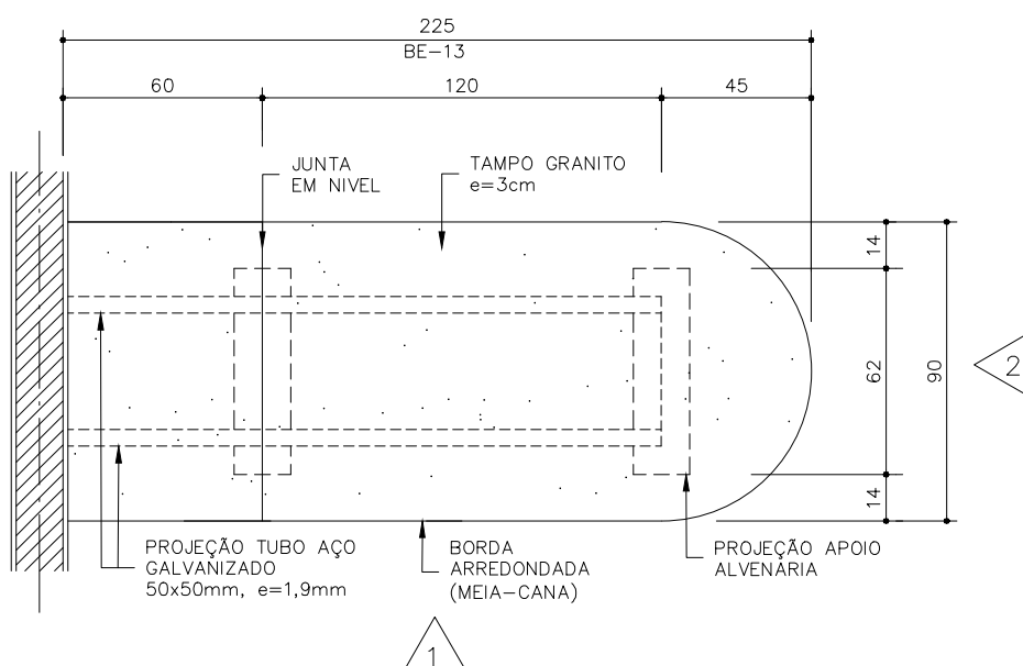
PLANTA TAMPO DA BANCADA ESCALA 1:25
