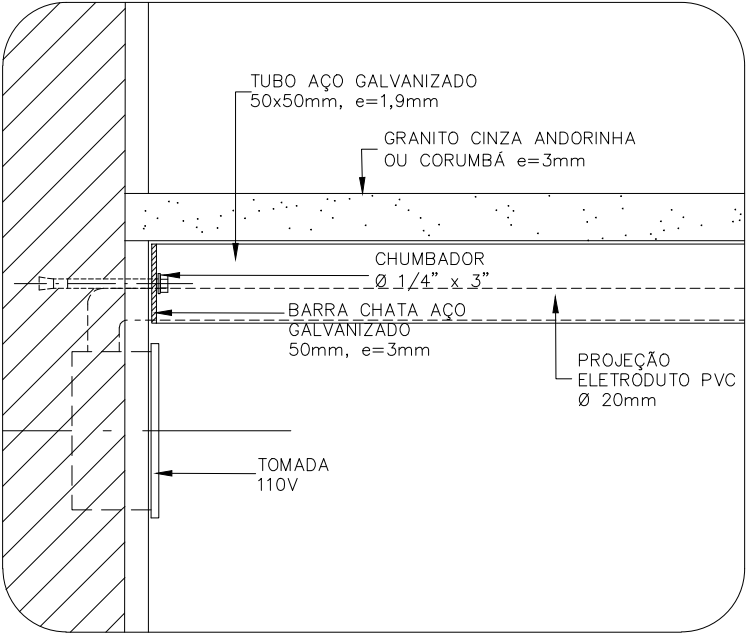
DETALHE 1 ESCALA 1:5
