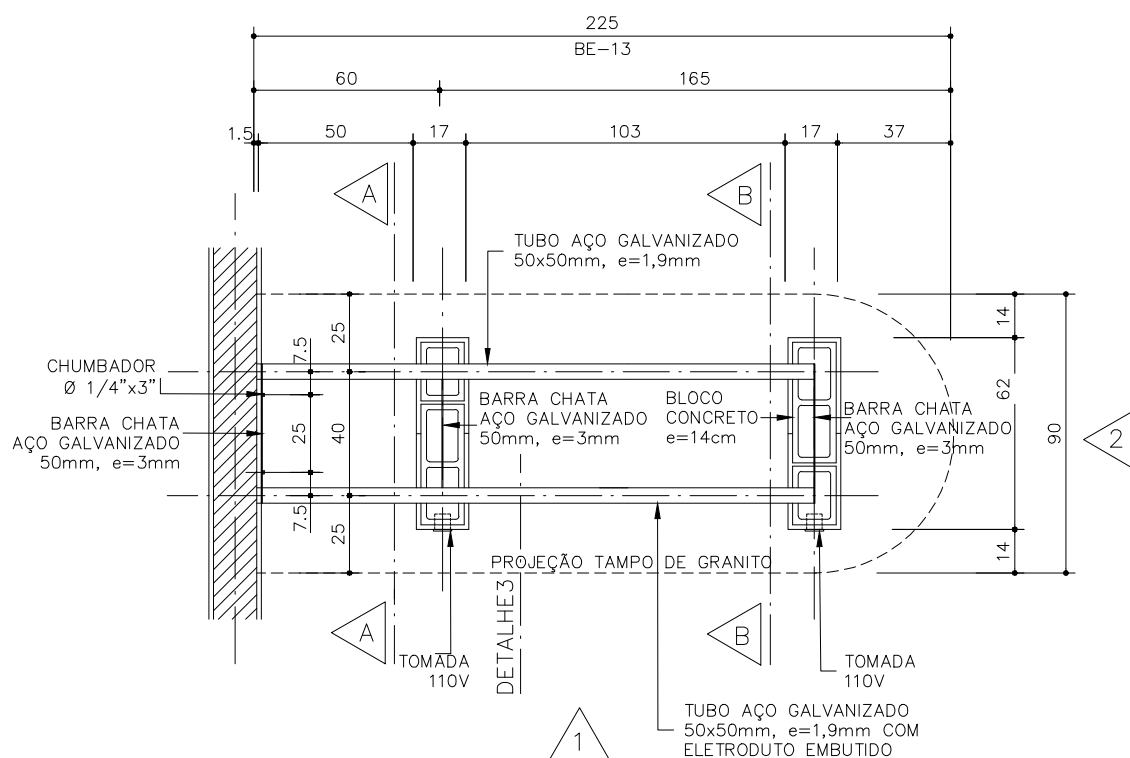
PLANTA BASE DE APOIOS
