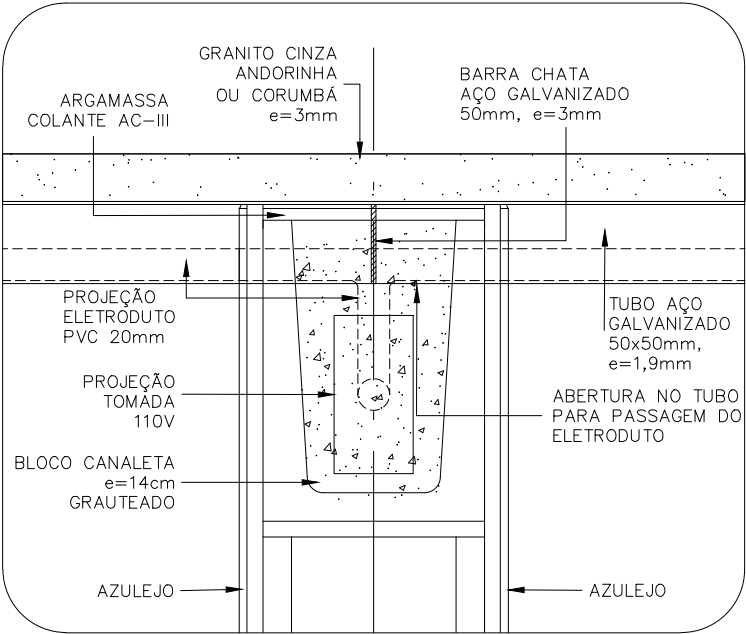
DETALHE 2 ESCALA 1:5
