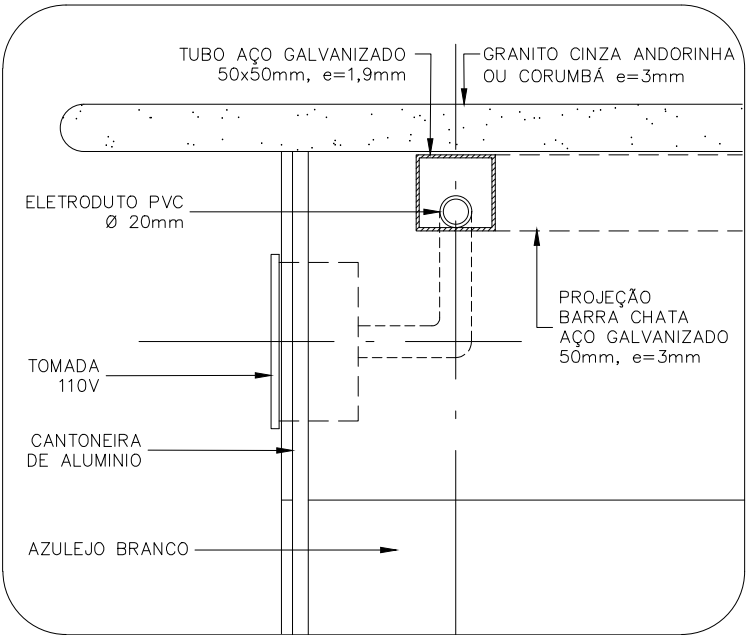
DETALHE 3 ESCALA 1:5
