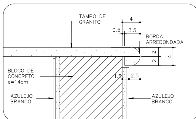
DETALHE 1 ESCALA 1:5
