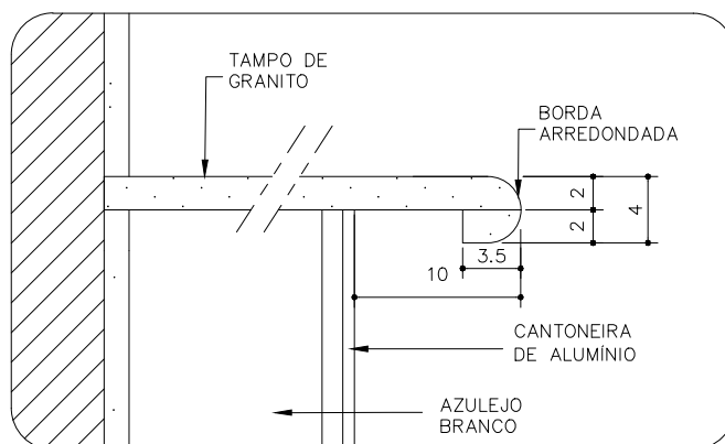
DETALHE 2 ESCALA 1:5
