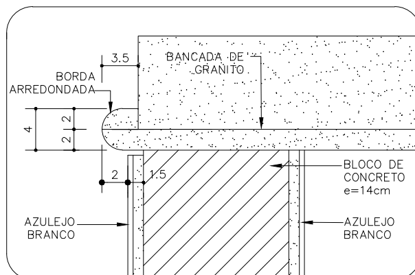
DETALHE 1 ESCALA 1:5
