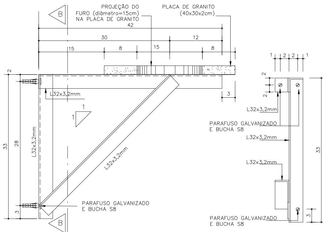
CORTE BB ESCALA 1:5
