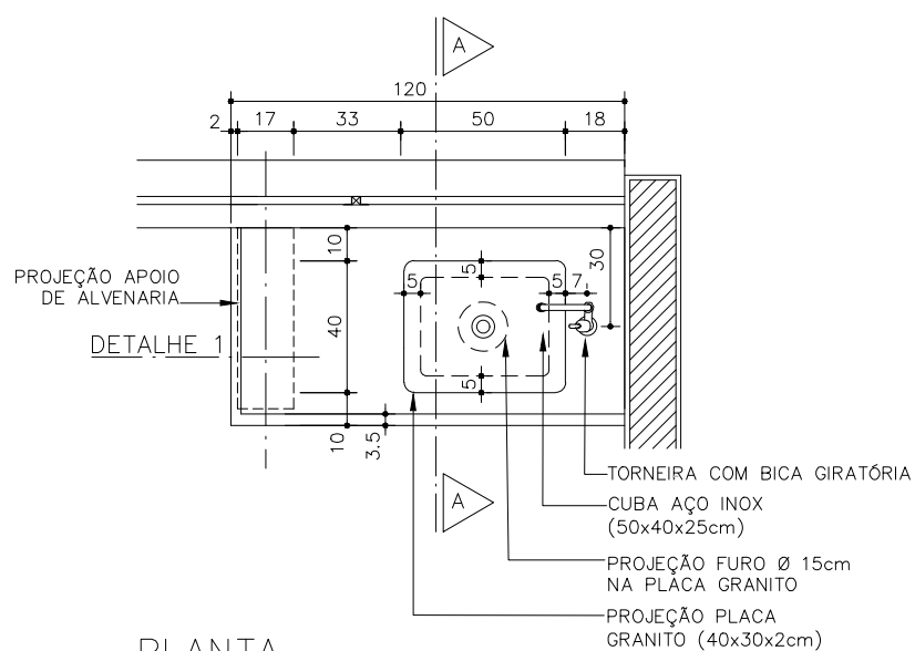
PLANTA ESCALA 1:25
