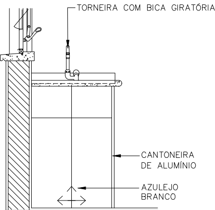
VISTA LATERAL ESCALA 1: 25
