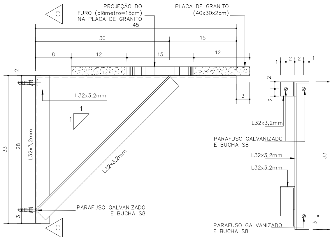
VISTA LATERAL
