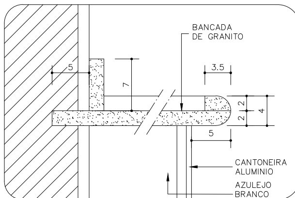
DETALHE 1
