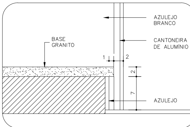
DETALHE 2
