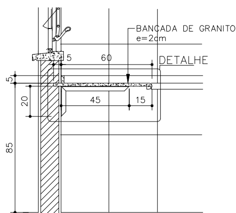
CORTE BB ESCALA 1:25
